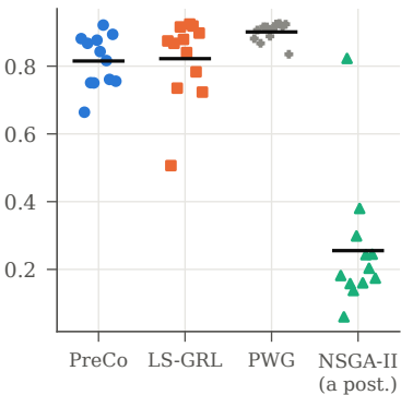
ASF regret
