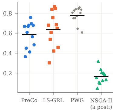
Weighted-sum regret
