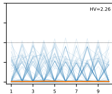
NSGA-III
