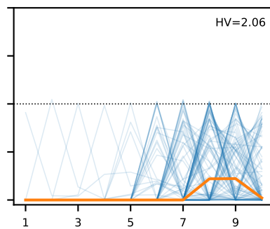
MaOEA-HAP
