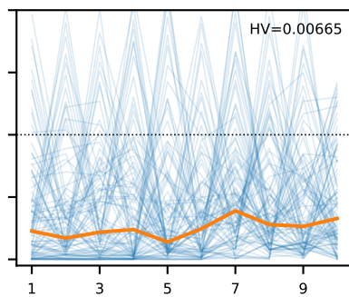
HLLDBEA fixed 0.10
