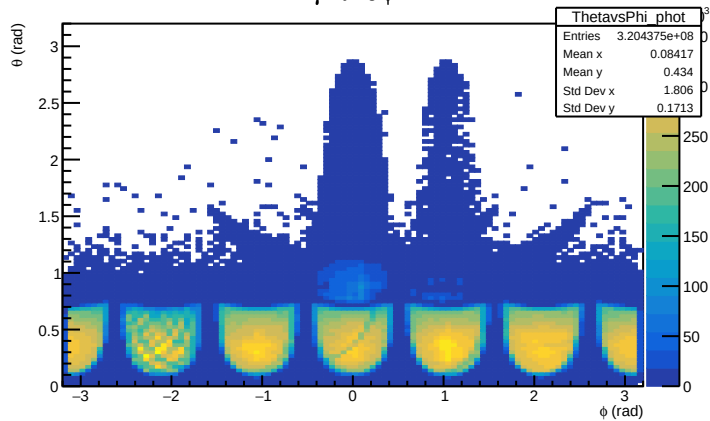
\gamma : \theta \text{ vs } \phi
