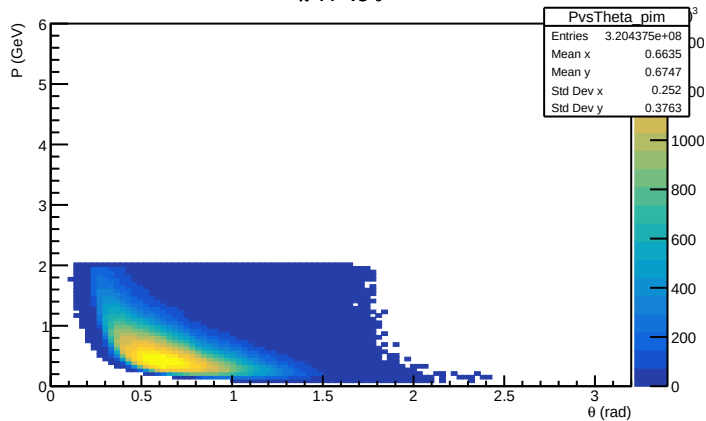
\pi^- : P \text{ vs } \theta
