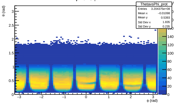
p^- : \theta \text{ vs } \phi
