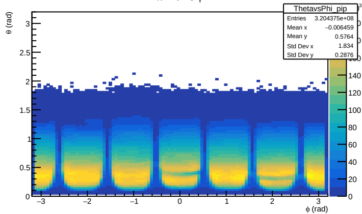
\pi^+ : \theta \text{ vs } \phi
