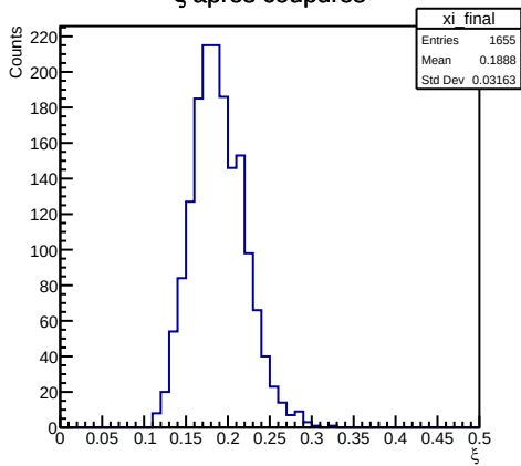
\xi apres coupures
