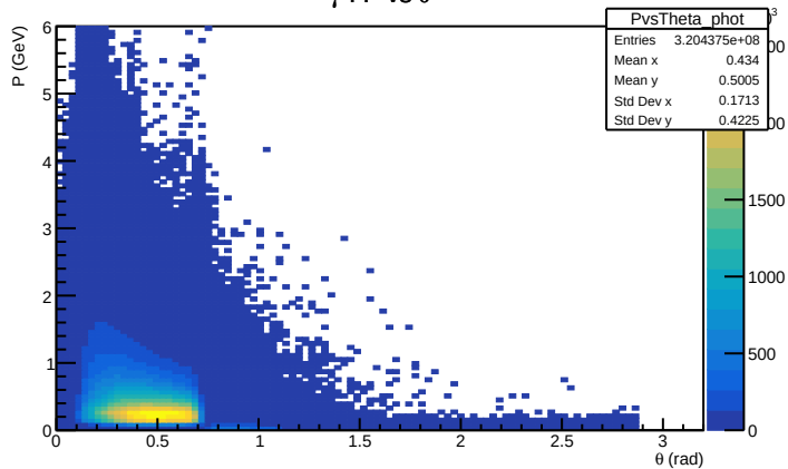
\gamma : P \text{ vs } \theta
