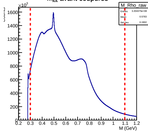
M_{\pi\pi} avant coupures
