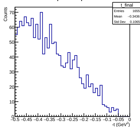
-t apres coupures
