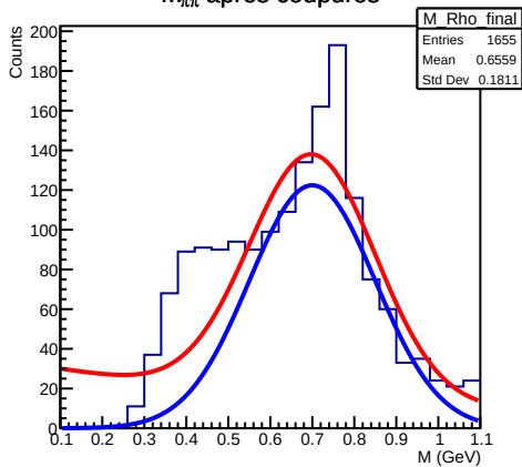
M_{\pi\pi} apres coupures
