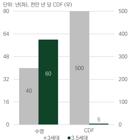
3세대·3.5세대 원자로 노형 비교
