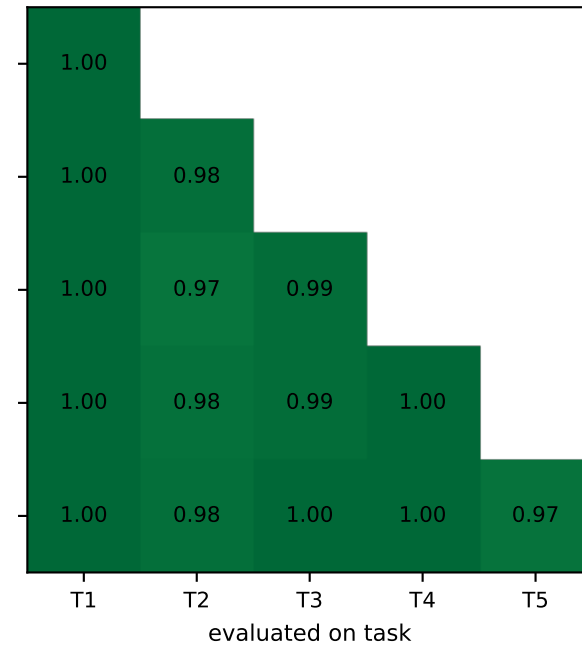
ALIF+SI+DM
