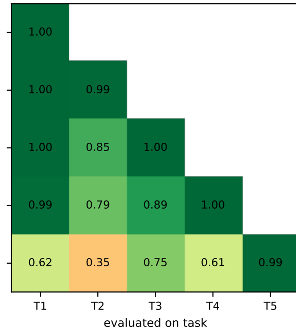
ALIF
