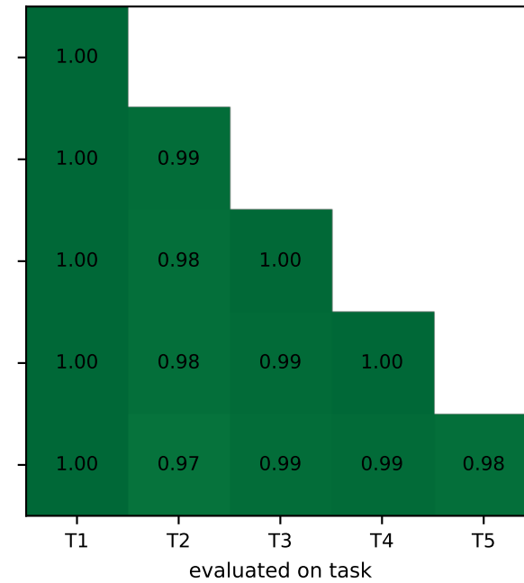
ALIF+SI
