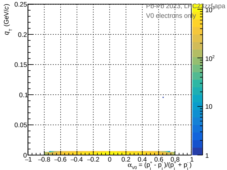
Armenteros-Podolanski - V0 electrons (fPidIndex=0)
