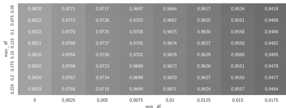
(б) Мультиномиальная модель, CountVectorizer
