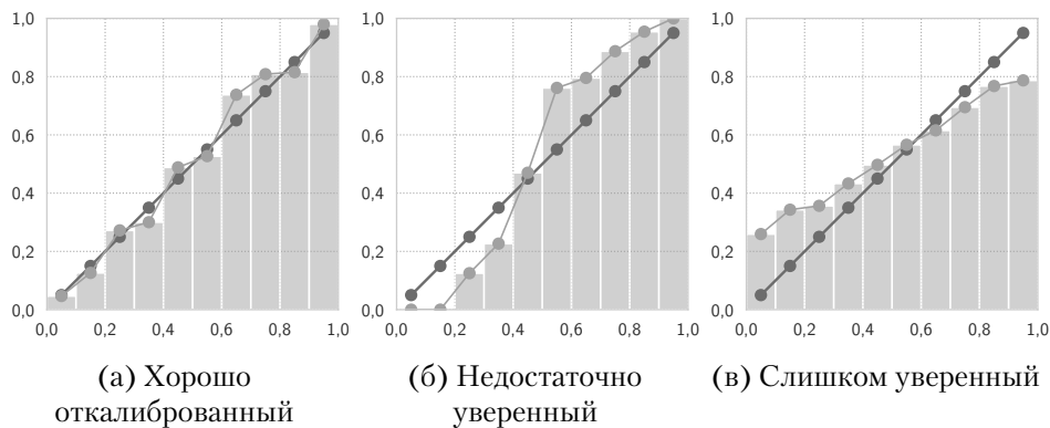
Рис. 5.17. Калибровка классификаторов: (а) хорошо откалиброванный классификатор, (б) недостаточно уверенный классификатор, (в) слишком уверенный классификатор
