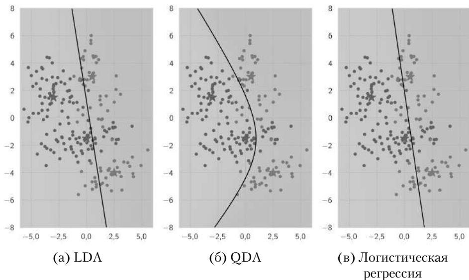
Рис. 5.19. Классификаторы, разделяющие две смеси гауссианов
