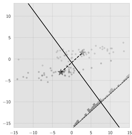
(б) Серединный перпендикуляр
