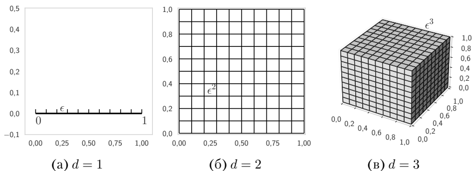
Рис. 6.4. Проклятие размерности: сетка с шагом \epsilon в разных размерностях
