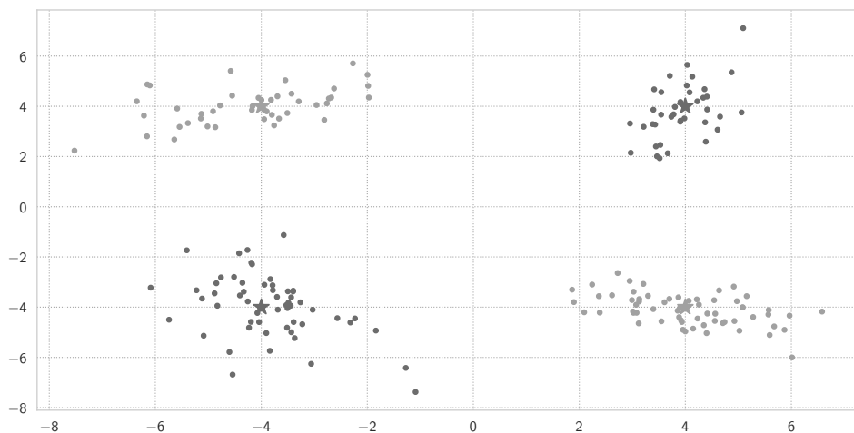
Рис. 1.8. Один перцептрон не сможет разделить точки этих двух классов, потому что не существует гиперплоскости (прямой), хорошо их разделяющей; но если разрешить провести две гиперплоскости, точки разделятся идеально
