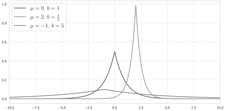
Рис. 4.32. Плотность распределения Лапласа p(w|\mu, b) = \frac{1}{2b}e^{-\frac{1}{b}|x-\mu|} для нескольких разных значений \mu и b
