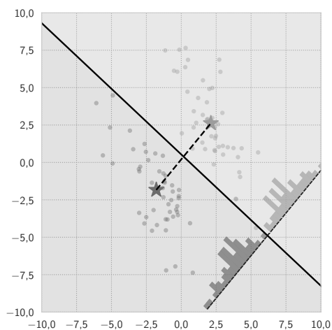
(а) Серединный перпендикуляр
