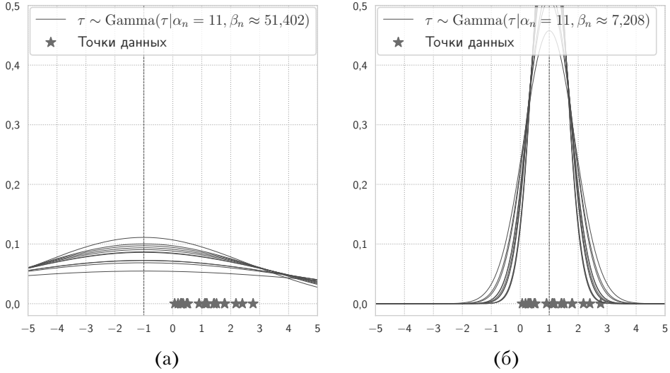
Рис. 6.16. Обучение гауссиана по \tau с двумя разными фиксированными \mu и априорным распределением \text{Gamma}(\tau | \alpha_0 = 1, \beta_0 = 1) : (а) выборка из апостериорного распределения для \mu = -1 ; (б) выборка из апостериорного распределения для \mu = 1
