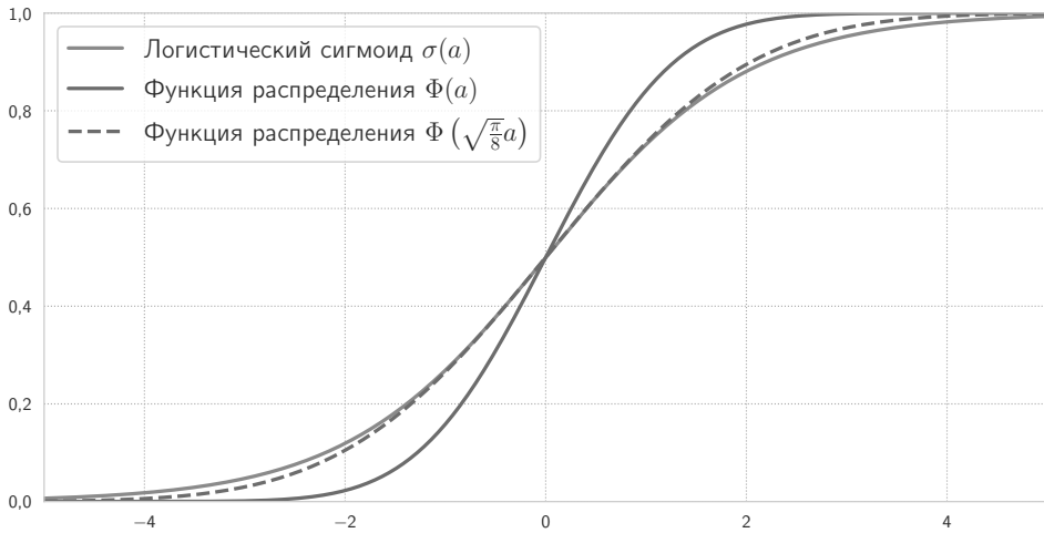
Рис. 5.9. Сравнение логистического сигмоида \sigma(a) и функции распределения стандартного гауссиана с подходящей нормировкой
