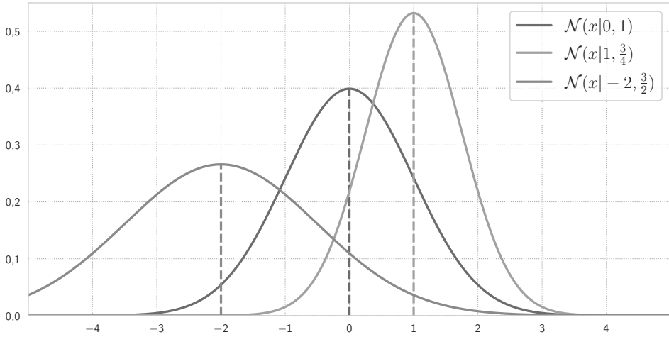
Рис. 3.8. Плотность одномерного нормального распределения с разными значениями \mu и \sigma
