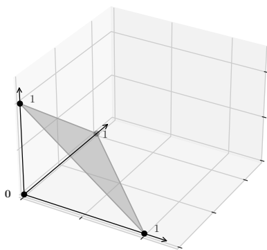
(б) двумерный симплекс
