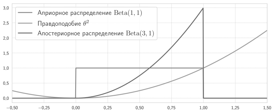
(а) Вероятность орла \theta , данные D с двумя орлами
