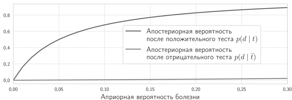
Рис. 2.6. Апостериорная вероятность p(d | t) как функция от априорной вероятности p(d) (превалентности) при фиксированных ошибках
