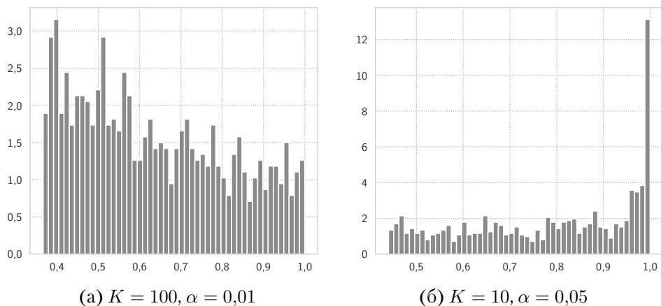
Рис. 2.18. Гистограммы значений наибольшего 1 % вероятностей для распределения Дирихле с \alpha = \alpha \cdot 1
