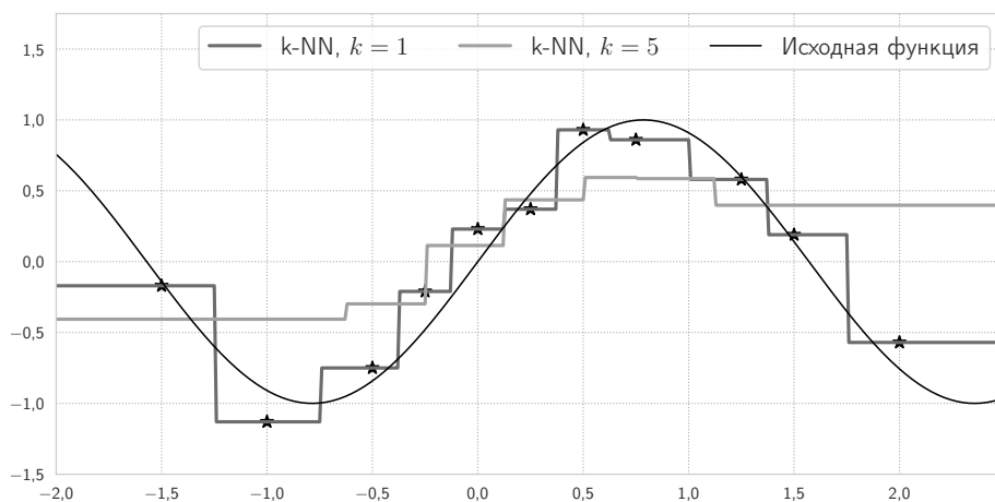
(а) 11 точек данных
