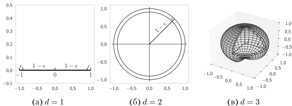
Рис. 6.5. Проклятие размерности: эффект кожуры апельсина толщины \epsilon в разных размерностях
