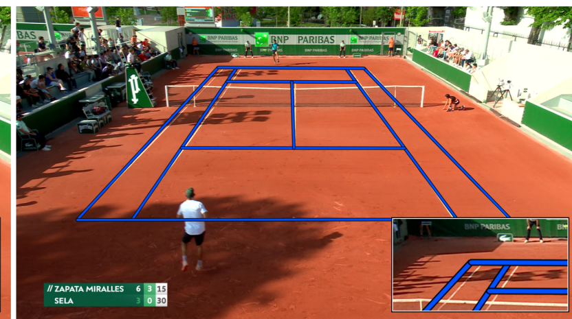
TVCalib
