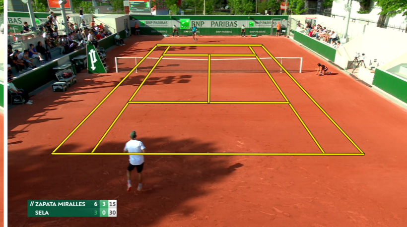
CourtAlign-E2E
