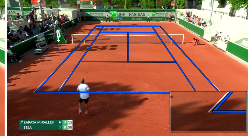
KpSFR
