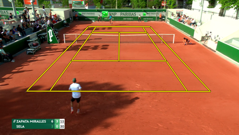
CourtAlign-2S
