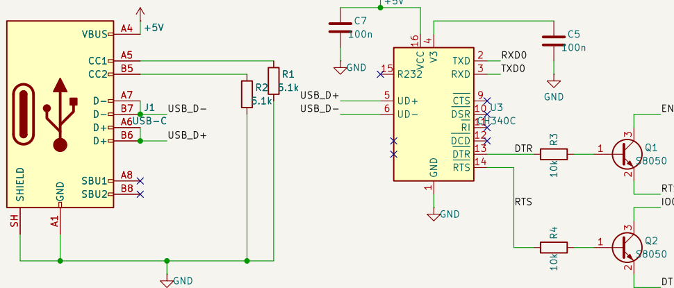
Auto-reset (DTR/RTS -> EN/I00, esptool style)
