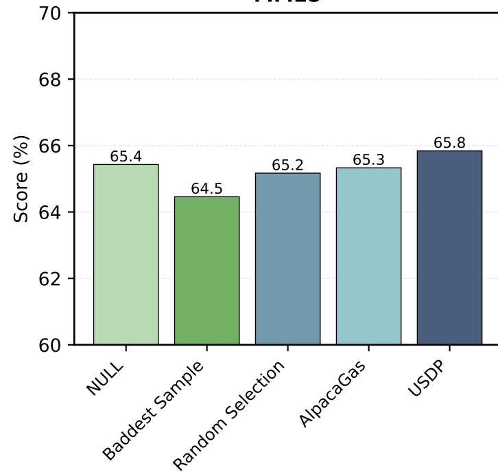
MMLU
