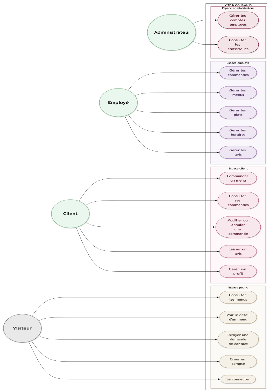
Figure 3 - Diagramme d'utilisation
