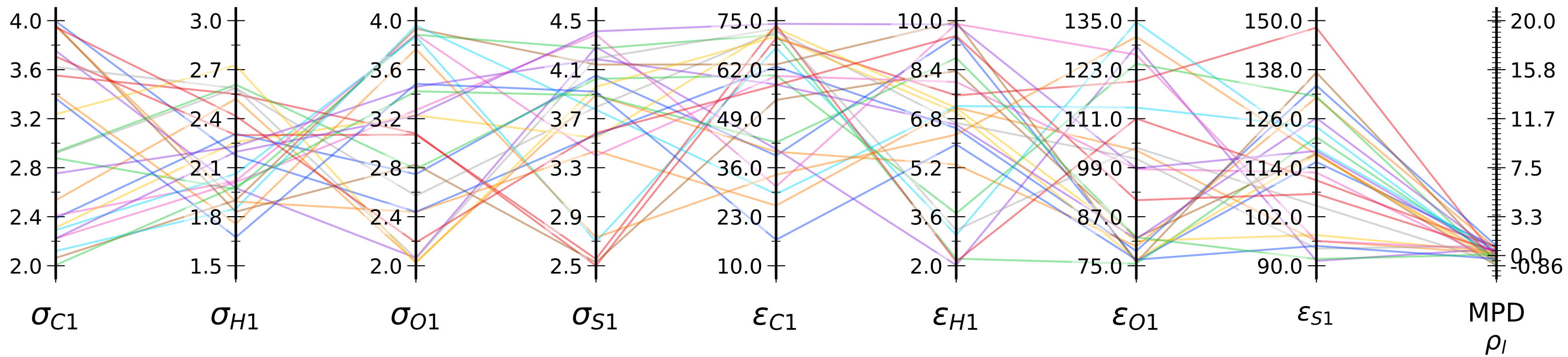
LJ Parameter Sets for DMSO LD Iters
