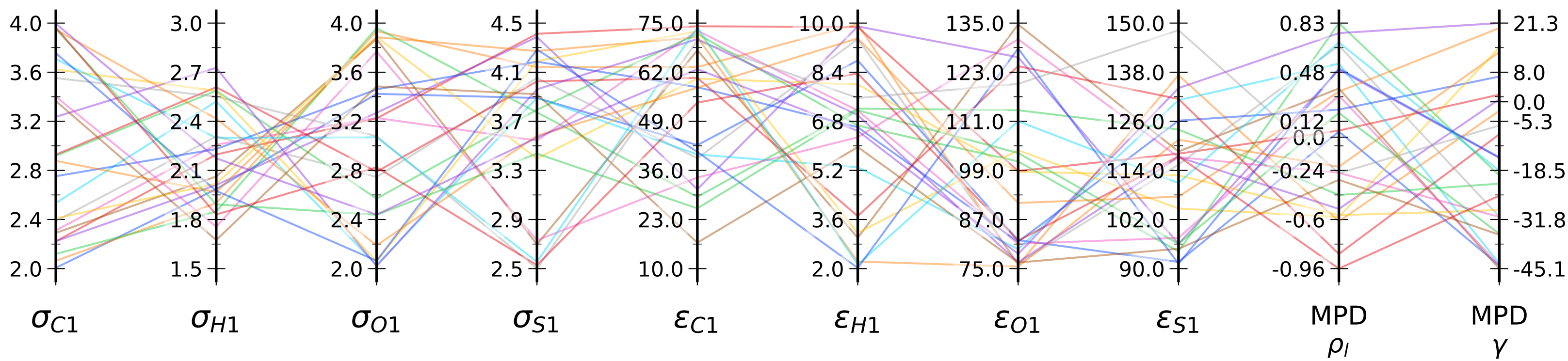
LJ Parameter Sets for DMSO ST Iter
