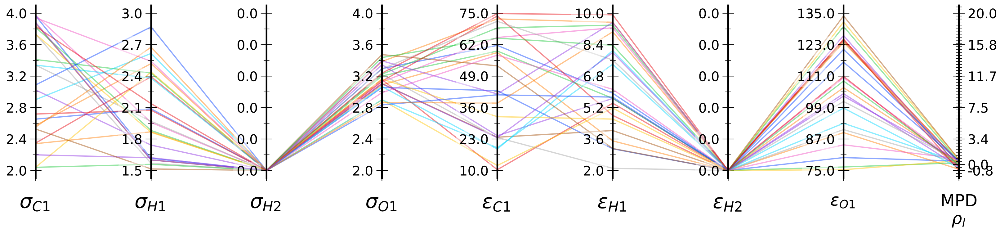
LJ Parameter Sets for EG LD Iters
