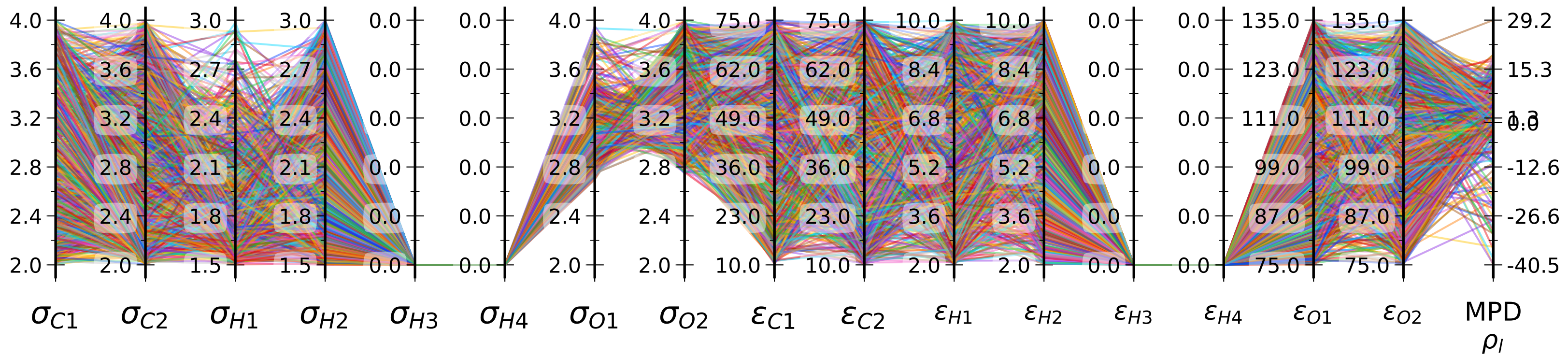
LJ Parameter Sets for Gly LD Iters
