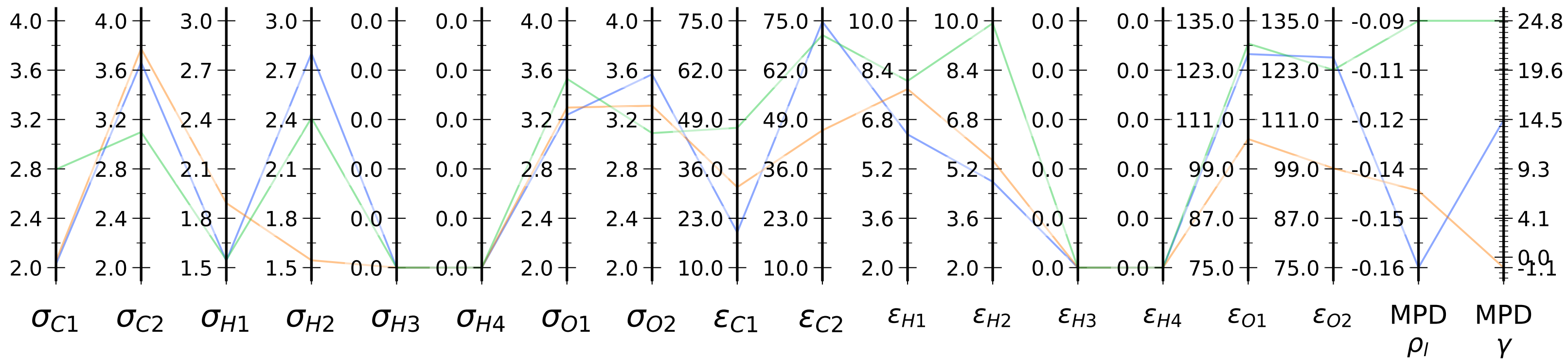
LJ Parameter Sets for Gly ST Iter
