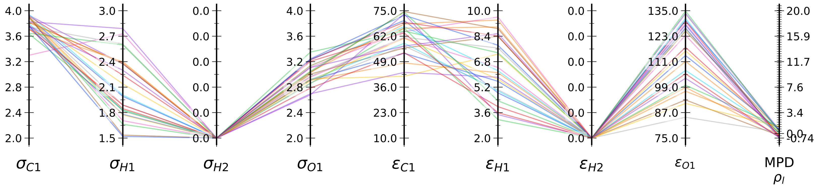
LJ Parameter Sets for MeOH LD Iters
