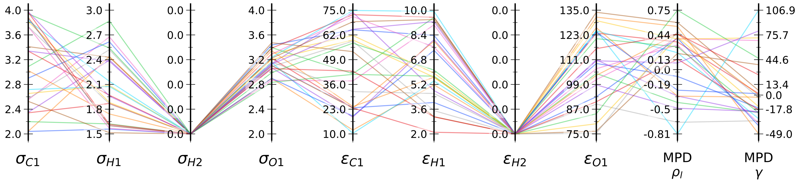
LJ Parameter Sets for EG ST Iter
