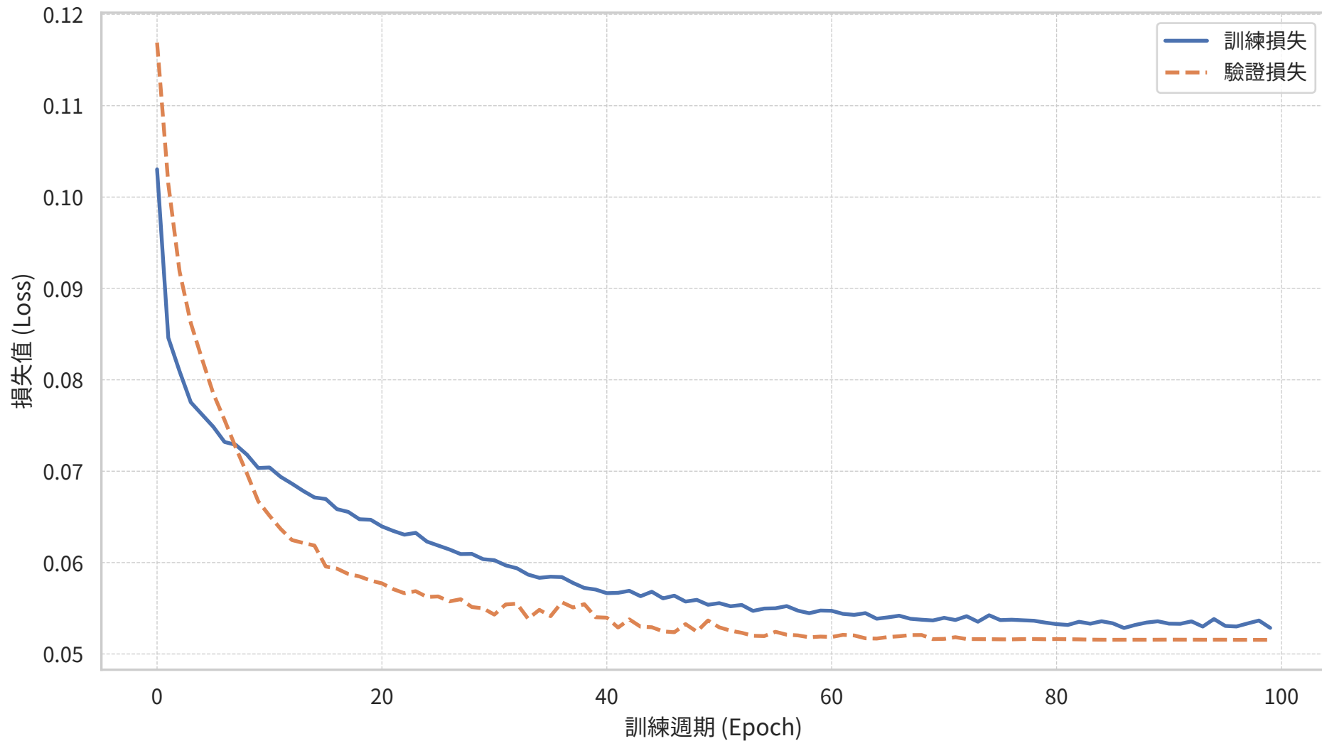
模型訓練過程損失曲線
