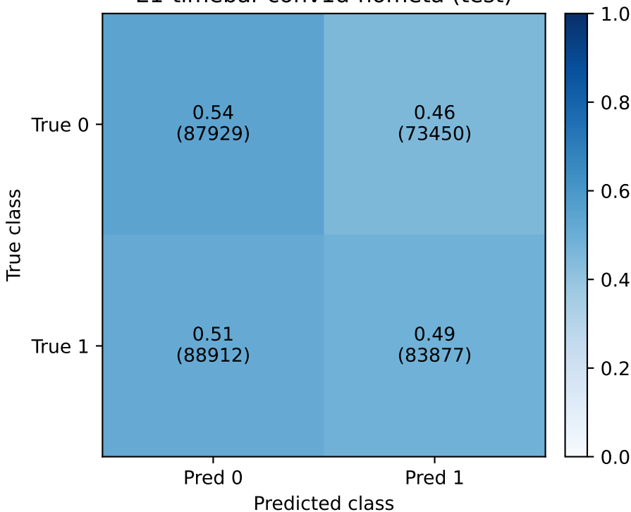
E1-timebar-conv1d-nometa (test)
