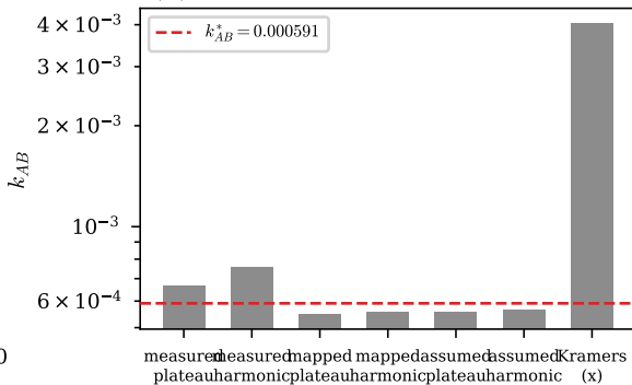
(d) Rate versus the exact reference
