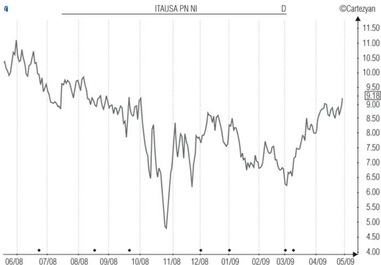
Gráfico 3.1 Gráfico de linha em Itausa PN usando apenas o preço de fechamento
