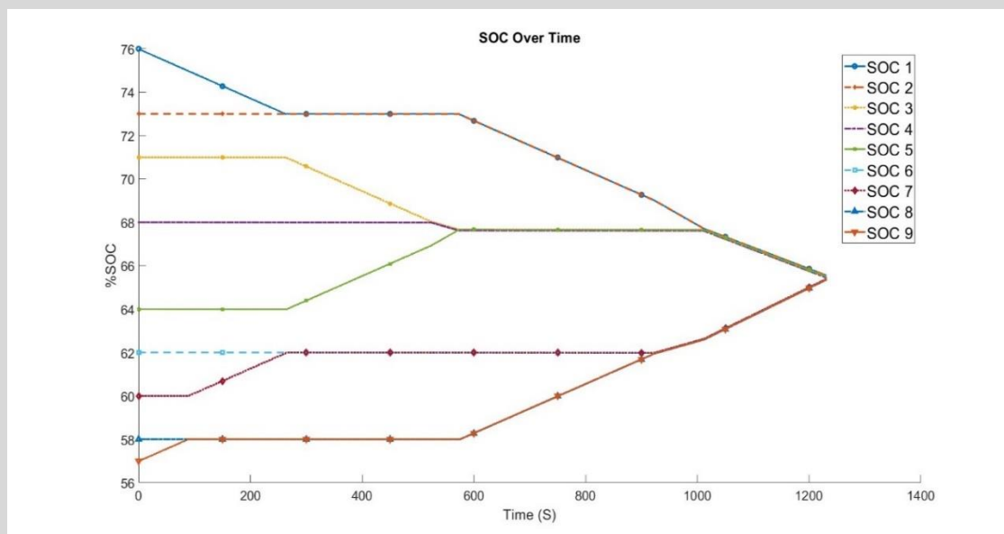
شکل ۴-۲۰ نمودار خروجی SOC باتری ها در فرآیند همسان سازی در روش پیشنهادی.
