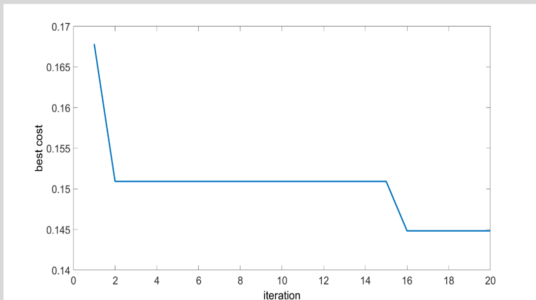
شکل ۴-۱۴ نمودار خروجی تابع هزینه به ازای ضرایب \alpha = \beta = \gamma = 0.33
