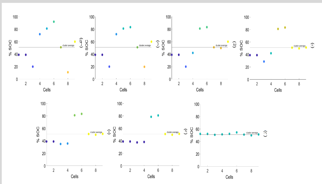
شکل ۴-۳ همسان سازی در هفت مرحله به ازای ضرایب \alpha = 0.1 و \beta = 0.8 ، \gamma = 0.1
