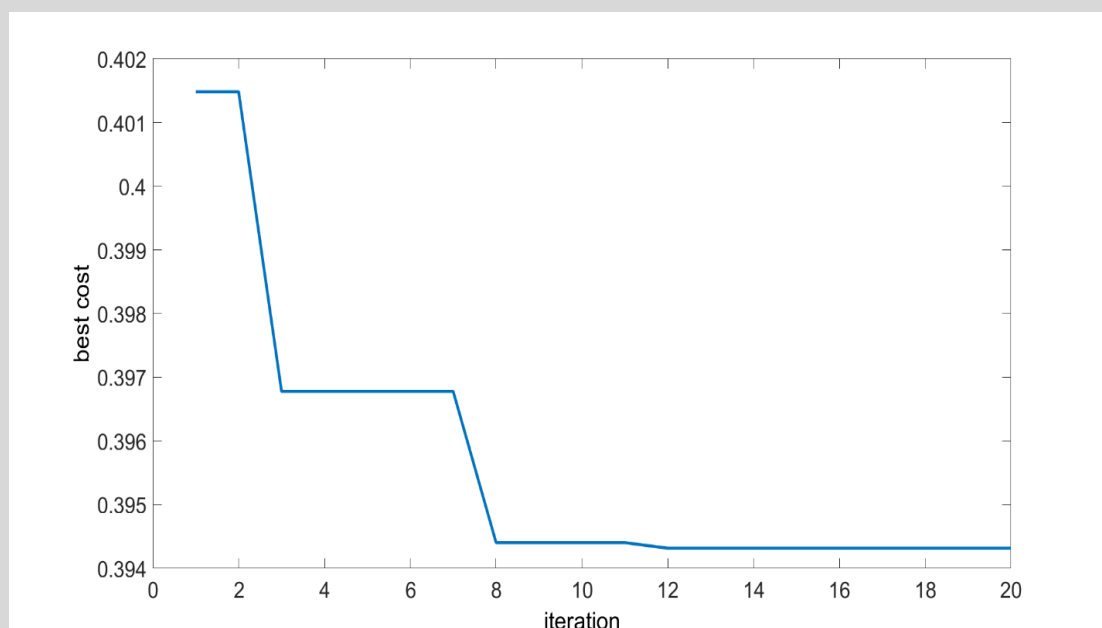
شکل ۴-۶ نمودار خروجی تابع هزینه به ازای ضرایب \alpha = 0.5 و \beta = 0.5 ، \gamma = 0 .
