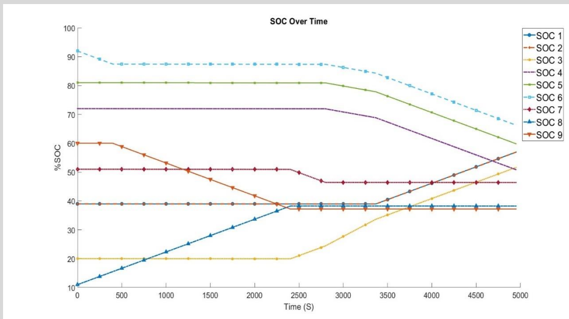
شکل ۴-۱۲ تغییرات وضعیت شارژ سلول‌ها در مراحل همسان‌سازی به ازای ضرایب \alpha = 0 و \beta = 0.5 ، \gamma = 0.5
