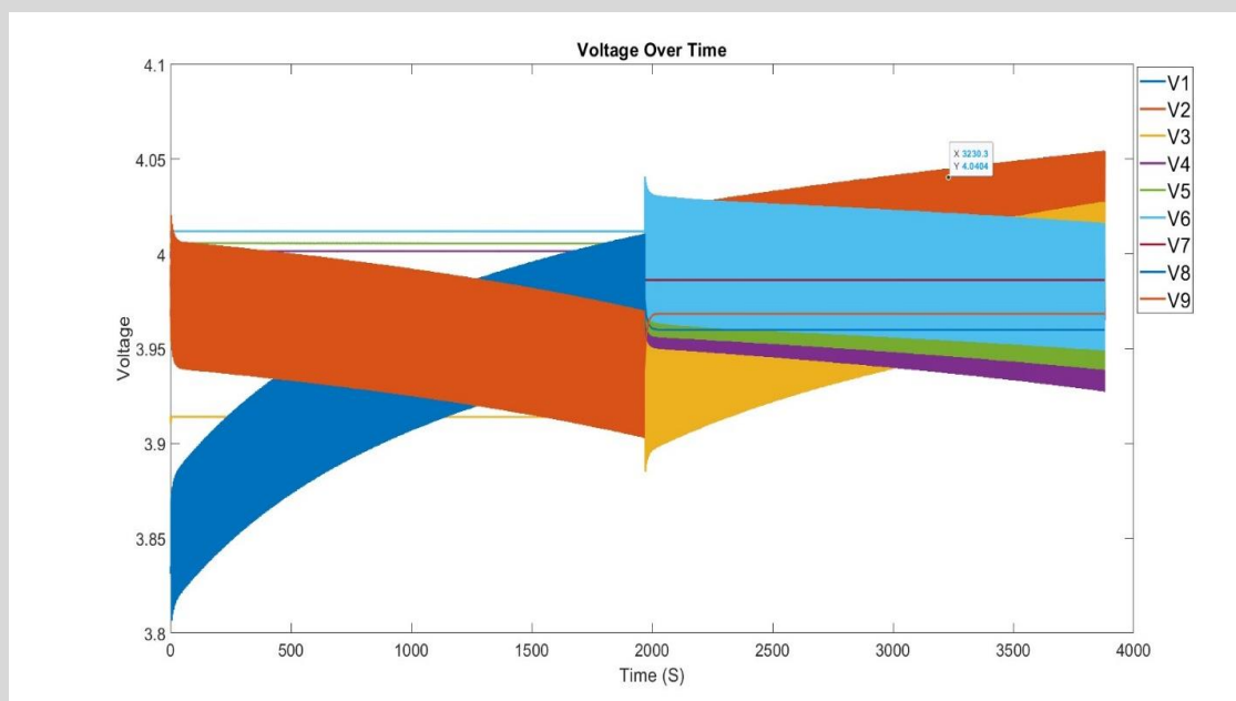
شکل ۴-۱۷ تغییرات ولتاژ سلول‌ها در فرآیند همسان‌سازی به ازای ضرایب \alpha = 0 و \beta = 0.5 ، \gamma = 0.5
