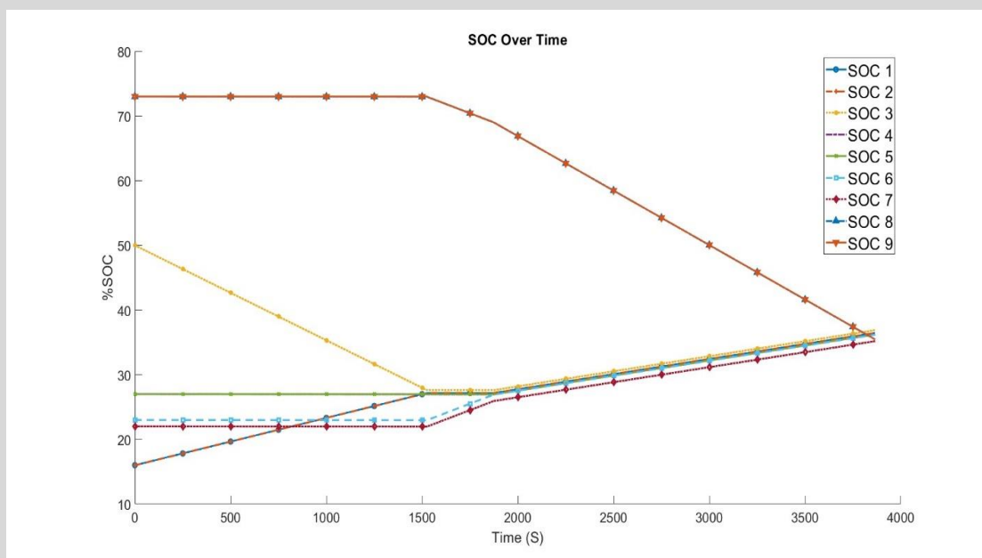
شکل ۴-۱۸ نمودار خروجی SOC باتری‌ها در فرآیند همسان‌سازی در روش پیشنهادی.
