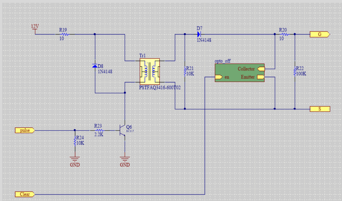
شکل ۳-۱۹ شماتیک گیت درایور ترانس پالسی.
