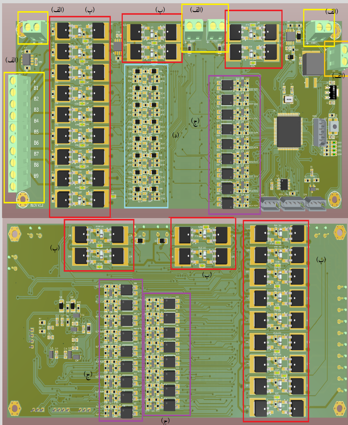
شکل ۳-۲۱ برد مدار چاپی مدار پیشنهادی شامل کانکتورها (الف)، سوئیچ‌های دوطرفه (ب)، گیت درایورهای اپتوکوپلری (ج) و گیت درایورهای ایزوله (د).
