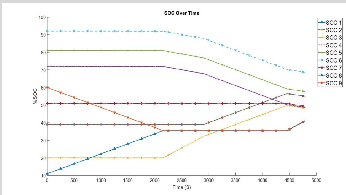
شکل ۴-۸ تغییرات وضعیت شارژ سلول‌ها در مراحل همسان‌سازی به ازای ضرایب \alpha = 0.5 و \beta = 0.5 ، \gamma = 0 .
