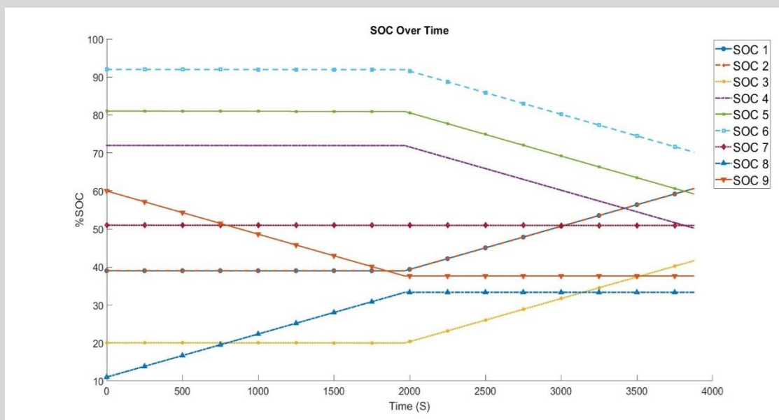
شکل ۴-۱۶ تغییرات وضعیت شارژ سلول‌ها در مراحل همسان‌سازی به ازای ضرایب \alpha = \beta = \gamma = 0.33
