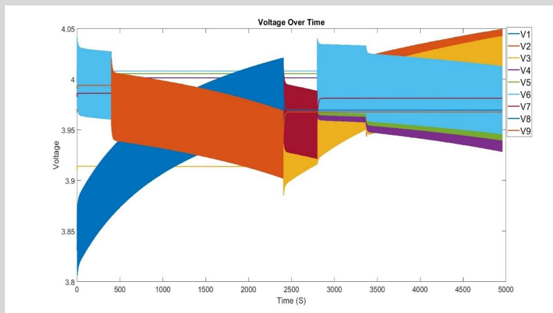
شکل ۴-۱۳ تغییرات ولتاژ سلول‌ها در فرآیند همسان‌سازی به ازای ضرایب \alpha = 0 و \beta = 0.5 ، \gamma = 0.5
