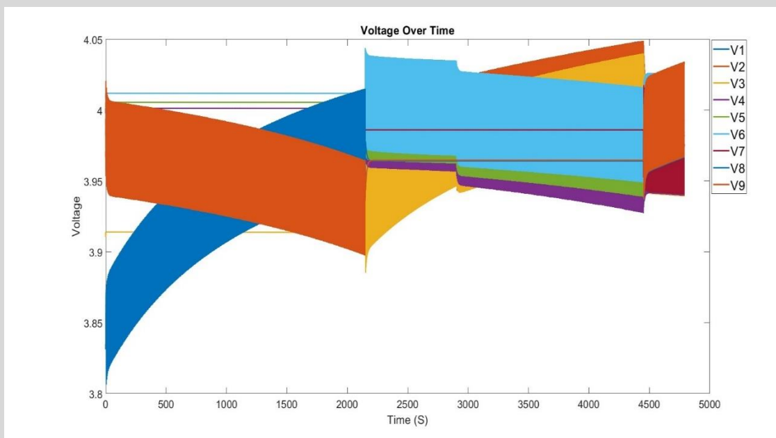
شکل ۴-۹ تغییرات ولتاژ سلول‌ها در فرآیند همسان‌سازی به ازای ضرایب \alpha = 0.5 و \beta = 0.5 ، \gamma = 0 .
