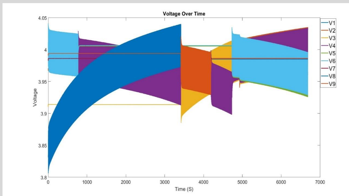
شکل ۴-۵ تغییرات ولتاژ سلول‌ها در فرآیند همسان‌سازی به ازای ضرایب \alpha = 0.1 و \beta = 0.8 ، \gamma = 0.1 .
