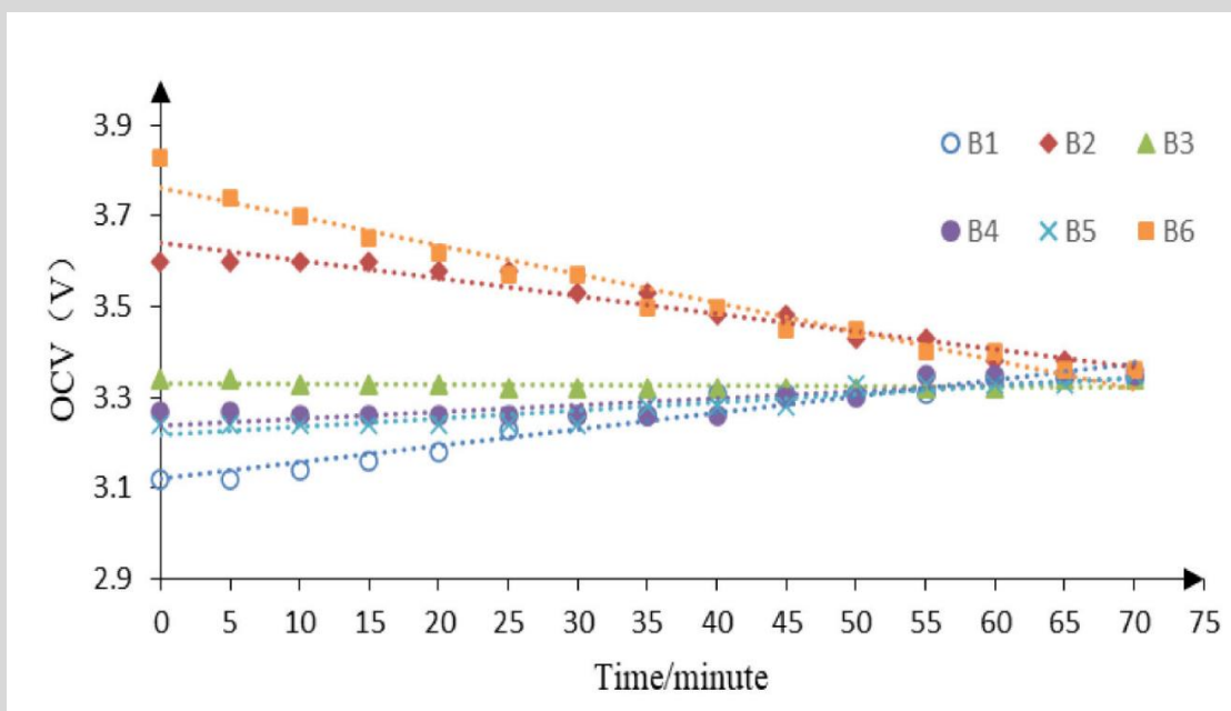
شکل ۴-۱۹ نمودار خروجی ولتاژ باتری‌ها در فرآیند همسان‌سازی با روش DBSCAN [۶۷].
