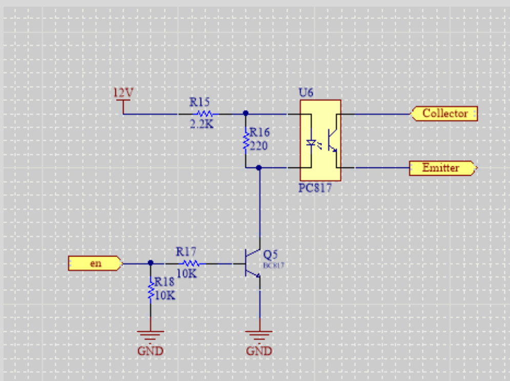
شکل ۳-۱۷ شماتیک گیت درایور ایتوکوپلری.
