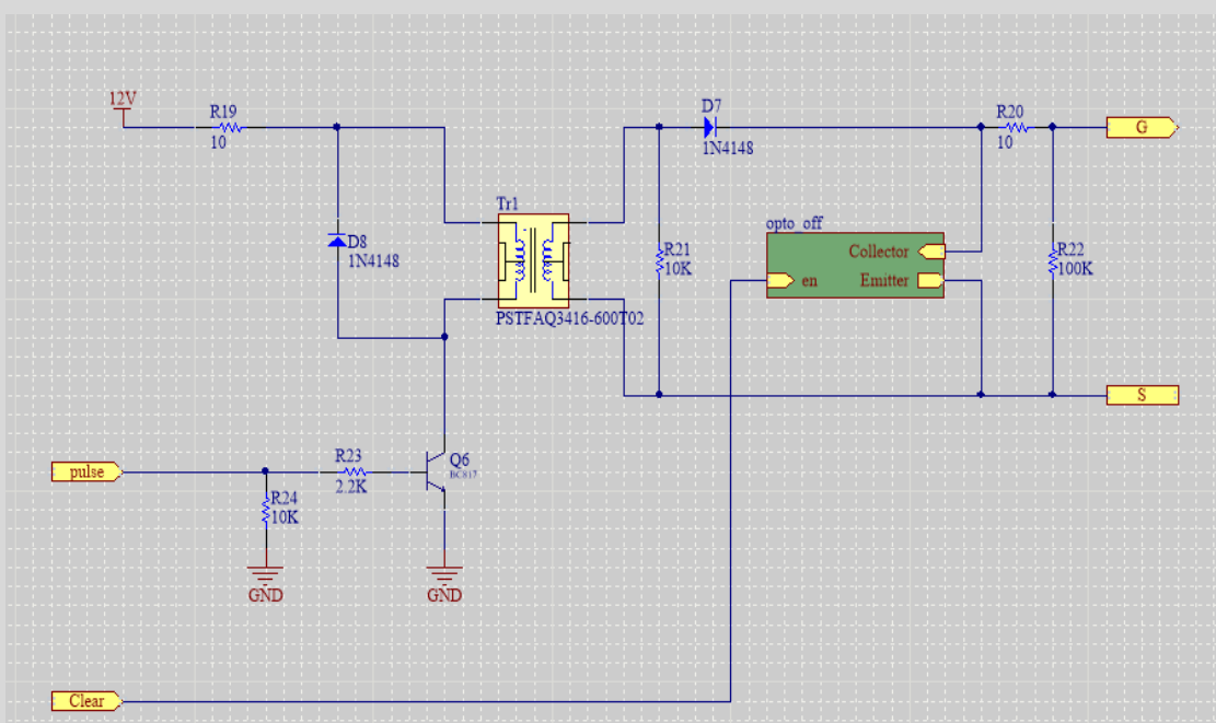
شکل ۱۹-۳ شماتیک گیت درایور ترانس پالسی.
