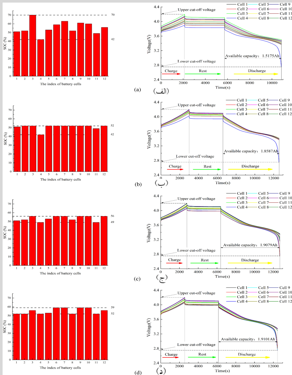
شکل ۲-۲۱ توزیع SOC و نتایج روش‌های همسان‌سازی. (الف) بدون همسان‌سازی (ب) روش آستانه ثابت
