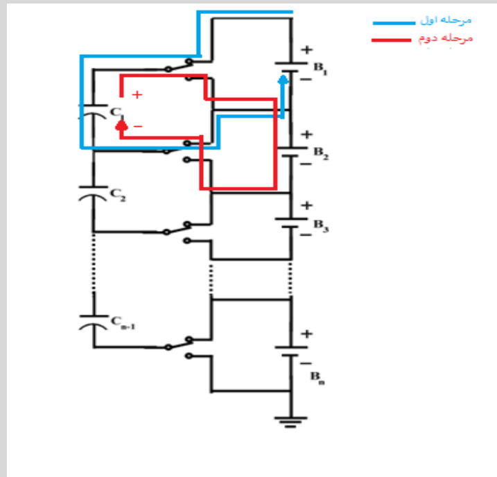
شکل ۲-۱۵ ساختار مدار همسان سازی بر مبنای سوئیچ خازنی [۵۳].
