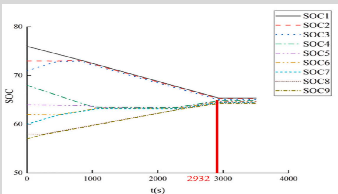
شکل ۴-۲۳ نمودار خروجی SOC باتری‌ها در فرآیند همسان‌سازی با روش FLC [۷۱].
