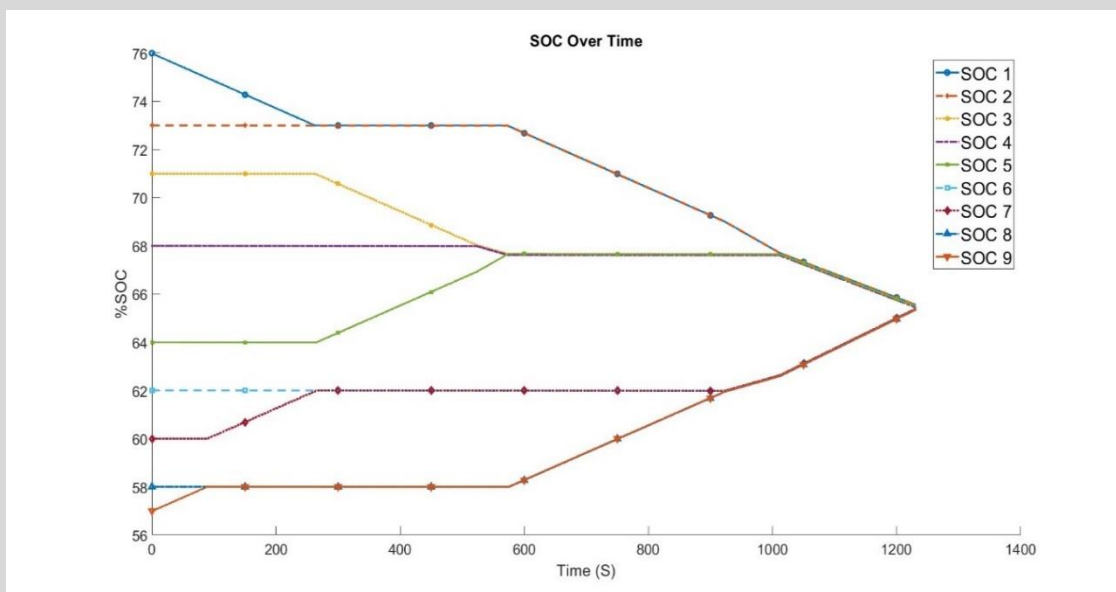
شکل ۴-۲۲ نمودار خروجی SOC باتری‌ها در فرآیند همسان‌سازی در روش پیشنهادی.
