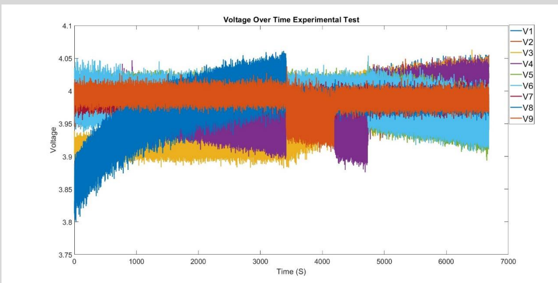
شکل ۴-۷ تغییرات ولتاژ سلول‌ها در فرآیند همسان‌سازی در عمل به ازای ضرایب \alpha = 0.1 و \beta = 0.8 ، \gamma = 0.1 .
