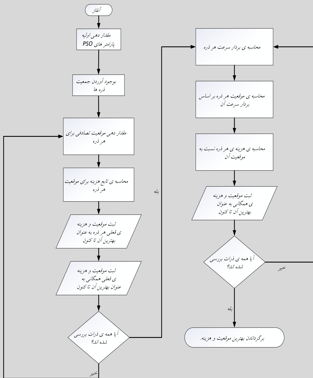
شکل ۱۱-۳ فلوچارت الگوریتم بهینه سازی \varepsilon بر اساس PSO.
