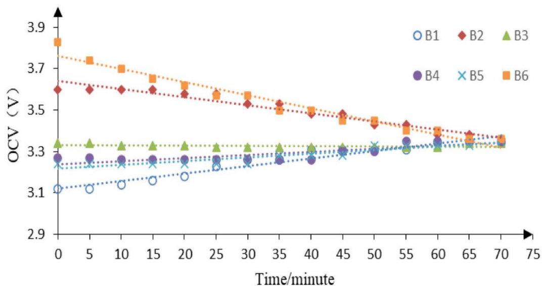
شکل ۴-۲۱ نمودار خروجی ولتاژ باتری‌ها در فرآیند همسان‌سازی با روش DBSCAN [۶۷].
