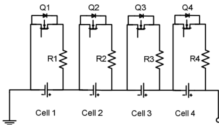
شکل ۲-۲ همسان‌ساز اتلافي با استفاده از مقاومت‌هاي شانت [۳۴].
