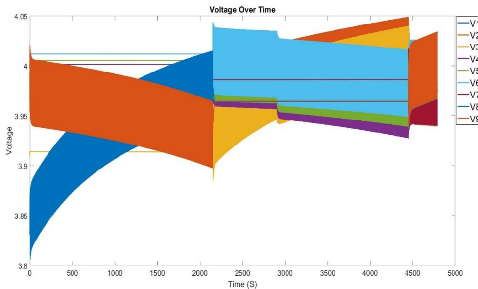
شکل ۴-۱۱ تغییرات ولتاژ سلول‌ها در فرآیند همسان‌سازی به ازای ضرایب \alpha = 0.5 و \beta = 0.5 و \gamma = 0 .
