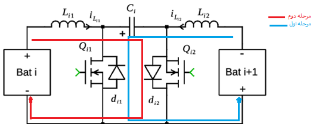
شکل ۱۳-۲ همسان‌ساز مبدل چوک [۵۴].
