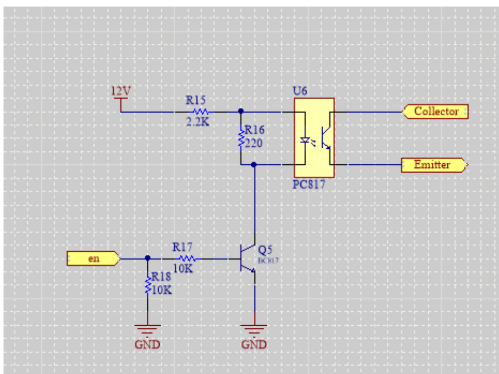
شکل ۳-۱۷ شماتیک گیت درایور ایتوکویلی.
