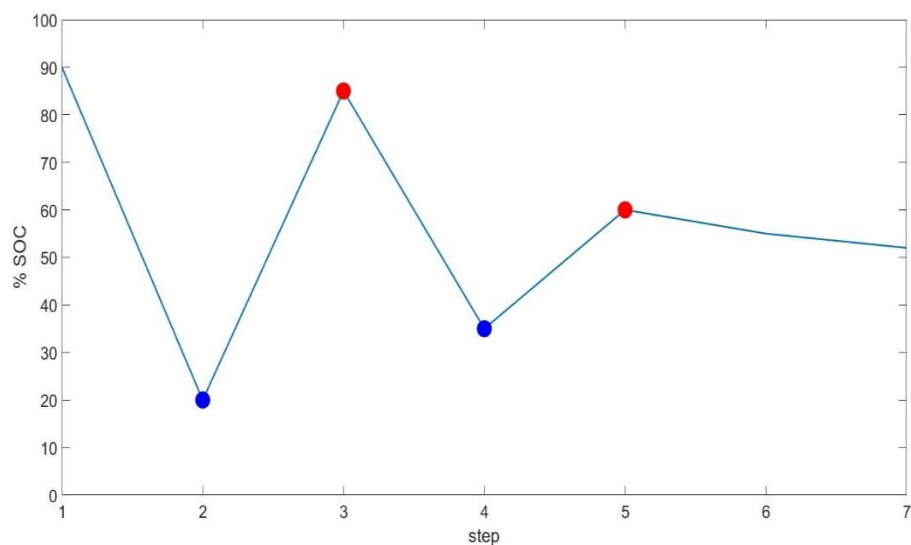
شکل ۳-۶ نمایشی از تغییرات SOC یک سلول در هر مرحله از همسان‌سازی که در آن محل قله‌ها و دره‌ها در فرآیند روی‌هم‌رفت مشخص شده است.
