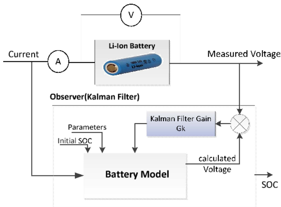
شکل ۱-۵ نمونه ساده از تخمین SOC توسط فیلتر کالمن [۲۳].
