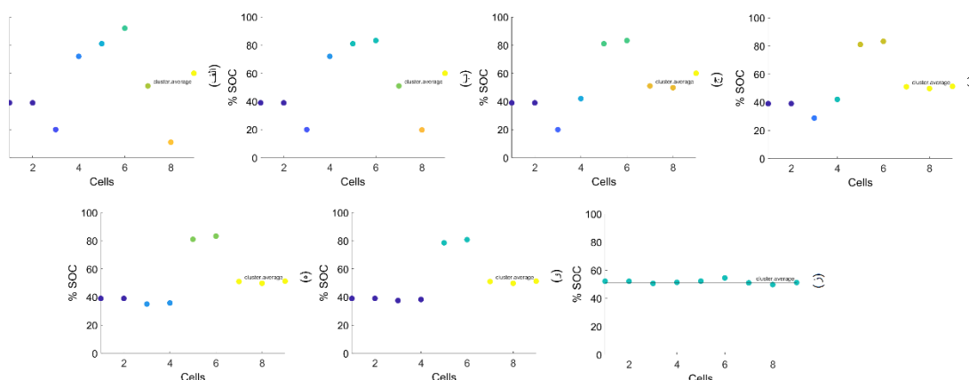
شکل ۳-۵ سلول‌های خوشه‌بندی شده با رنگ‌های یکسان، همراه با مراحل همسان‌سازی سلول‌ها (الف) و نتیجه‌ی به دست آمده (ز) در ازای \varepsilon = 2/16 .
