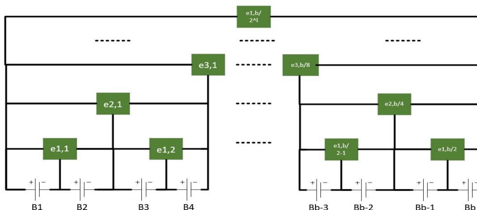
شکل ۹-۲ نمایی از انتقال سریالی سلول به سلول لایه‌ای.
