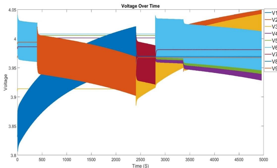
شکل ۴-۱۵ تغییرات ولتاژ سلول‌ها در فرآیند همسان‌سازی به ازای ضرایب \alpha = 0 و \beta = 0.5 ، \gamma = 0.5
