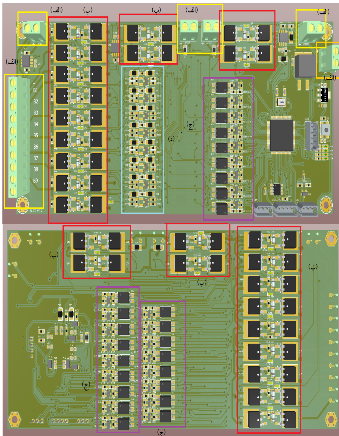
شکل ۳-۲۱ برد مدار چاپی مدار پیشنهادی شامل کانکتورها (الف)، سوئیچ‌های دوطرفه (ب)، گیت درایورهای ایتوکوپلری (ج) و گیت درایورهای ایزوله (د).
