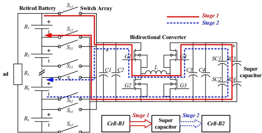
شکل ۲۳-۲ نمایی از فرآیند انتقال شارژ گروه به گروه [۶۷].
