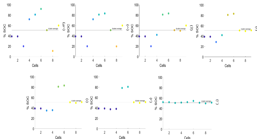
شکل ۳-۴ همسان سازی در هفت مرحله به ازای ضرایب \alpha = 0.1 و \beta = 0.8 ، \gamma = 0.1
