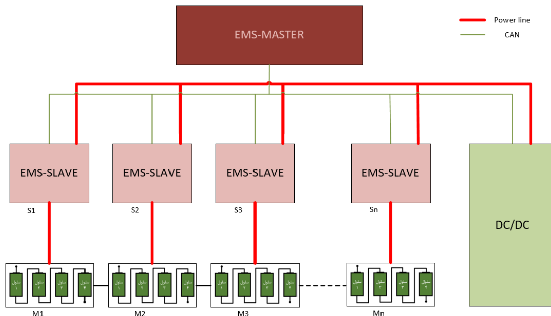
شکل ۳-۲ نحوه پیکربندی سیستم همسان‌سازی پیشنهادی خودرو.
