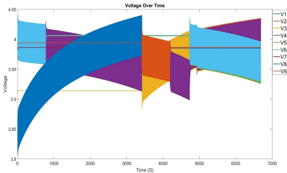
شکل ۴-۶ تغییرات ولتاژ سلول‌ها در فرآیند همسان‌سازی به ازای ضرایب \alpha = 0.1 و \beta = 0.8 ، \gamma = 0.1 .
