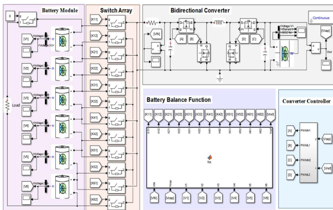
شکل ۲-۲۵ مدل شبیه‌سازی شده همسان‌ساز در مطلب [۶۷].
