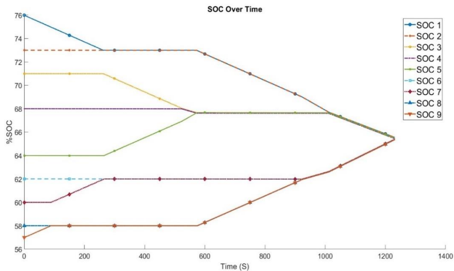
شکل ۴-۲۲ نمودار خروجی SOC باتری‌ها در فرآیند همسان‌سازی در روش پیشنهادی.
