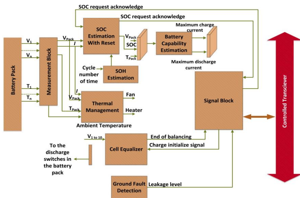
شکل ۱-۱ نمایی کلی از یک سیستم مدیریت باتری [۱۱].
