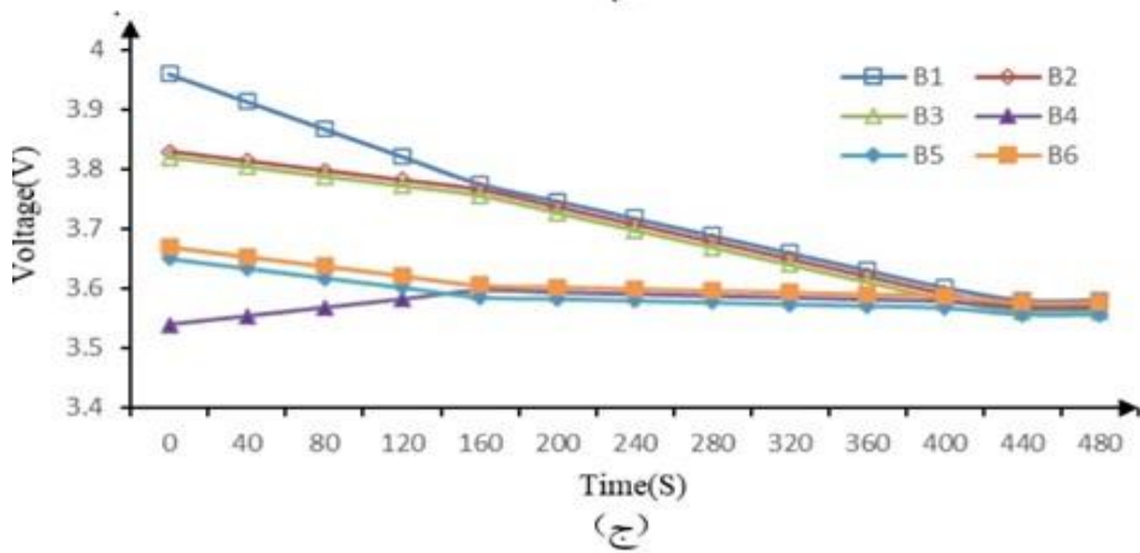
شکل ۲-۲۷ وضعیت باتری در شرایط مختلف تعادل در پیاده‌سازی عملی (الف) وضعیت باتری در حالت تعادل در ایستا. (ب) وضعیت باتری در حالت تعادل در شارژ. (ج) وضعیت باتری در حالت تعادل در دشارژ [۶۷].
