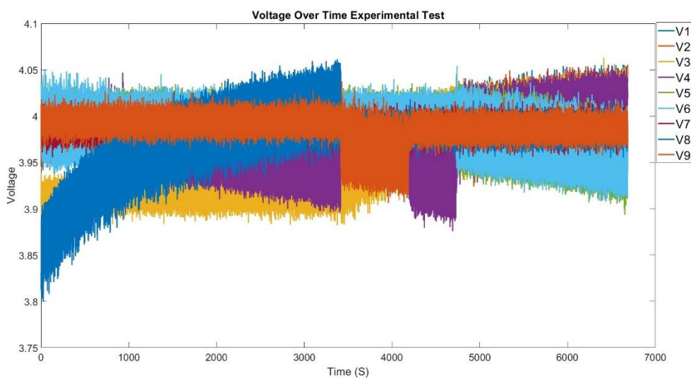
شکل ۴-۷ تغییرات ولتاژ سلول‌ها در فرآیند همسان‌سازی در عمل به ازای ضرایب \alpha = 0.1 و \beta = 0.8 ، \gamma = 0.1 .
