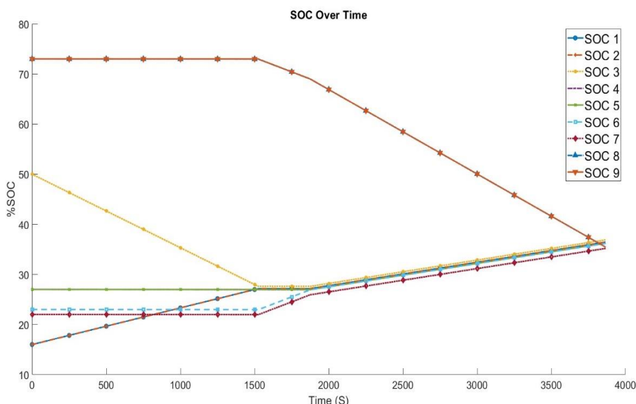
شکل ۴-۲۰ نمودار خروجی SOC باتری‌ها در فرآیند همسان‌سازی در روش پیشنهادی.
