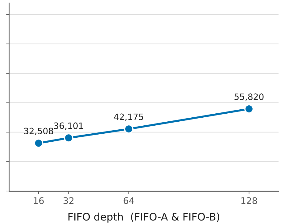
LUT vs FIFO_D
