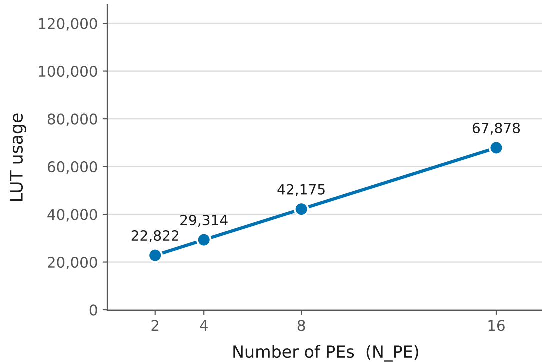
LUT vs N_PE
