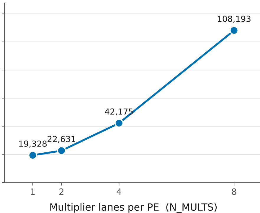
LUT vs N_MULTS
