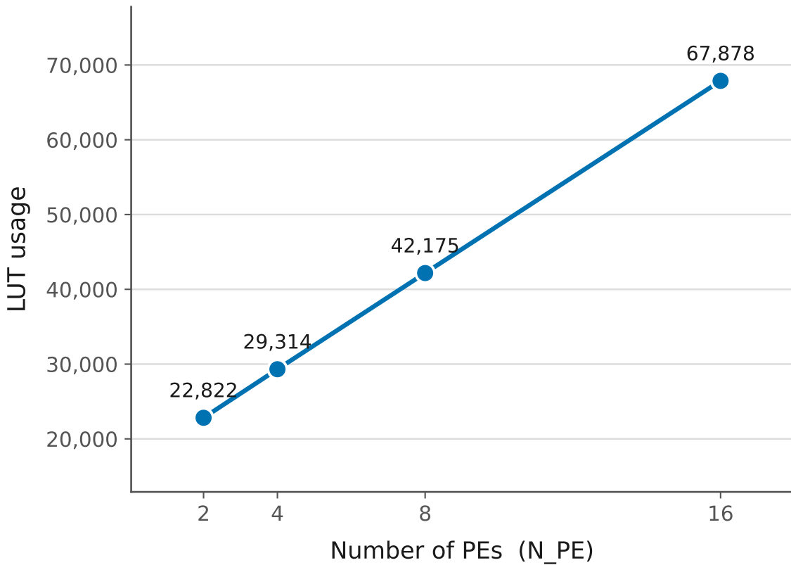
LUT usage vs N_PE
