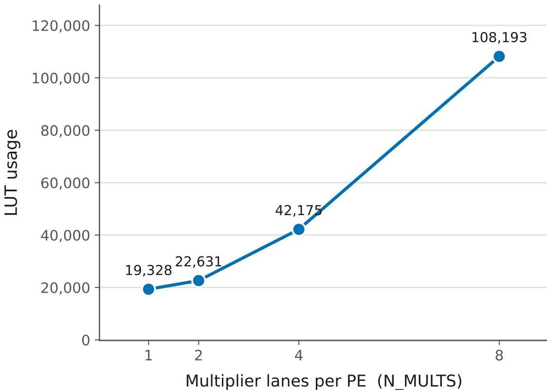
LUT usage vs N_MULTS
