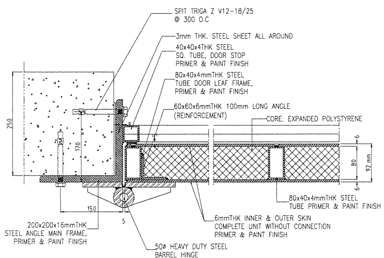
DETAIL-A SCALE: 1:3
