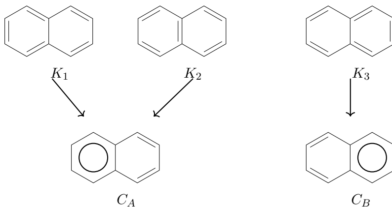
FIGURE 6 – Les deux couvertures de Clar du naphtalène
