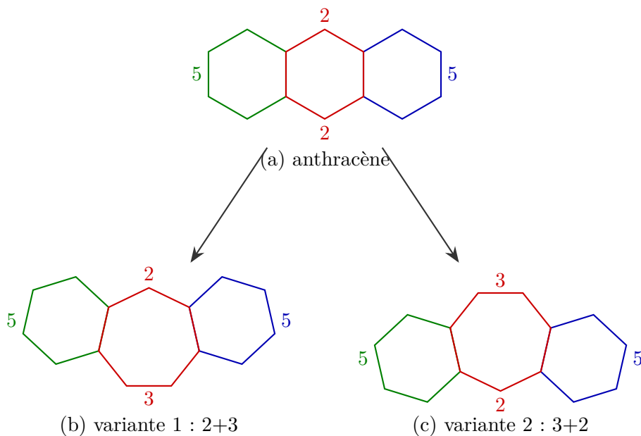
FIGURE 9 – Anthracène et transformation du cycle central en heptagone.
