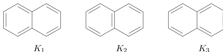
FIGURE 4 – Les trois structures de Kekulé du naphthalène.
