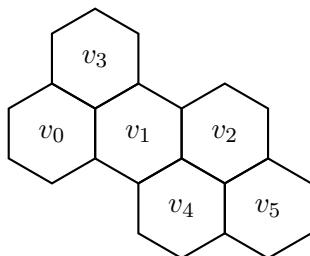
FIGURE 2 – Un benzénoïde non linéaire à six hexagones (v_0, \dots, v_5) .
