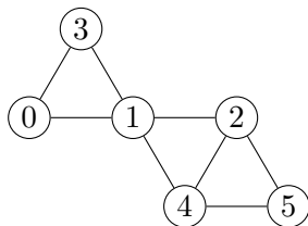
FIGURE 3 – Graphe dual G_D du benzénoïde de la figure ??.
