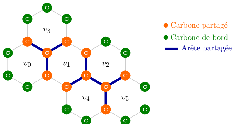
FIGURE 9 – Mise en évidence des carbones et des arêtes partagés
