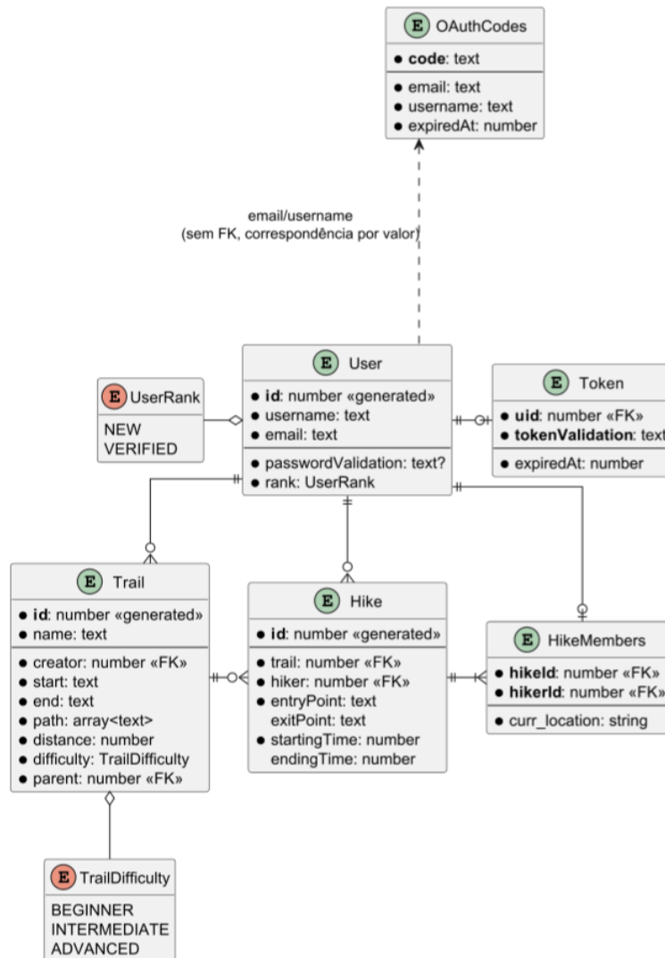
Figura 4.10: UML do Modelo ER desenvolvido
