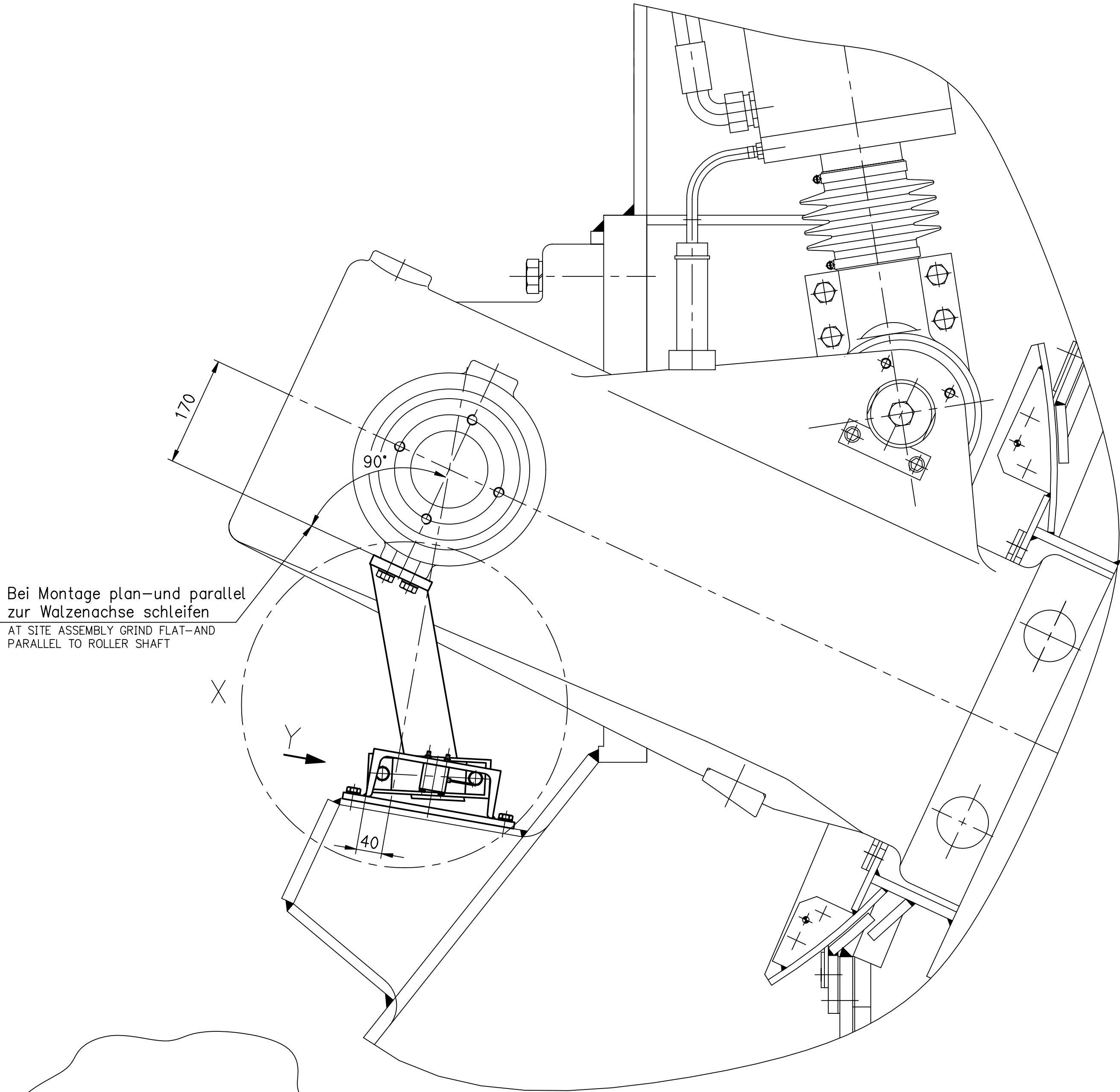
Ansicht Y VIEW 1:2
