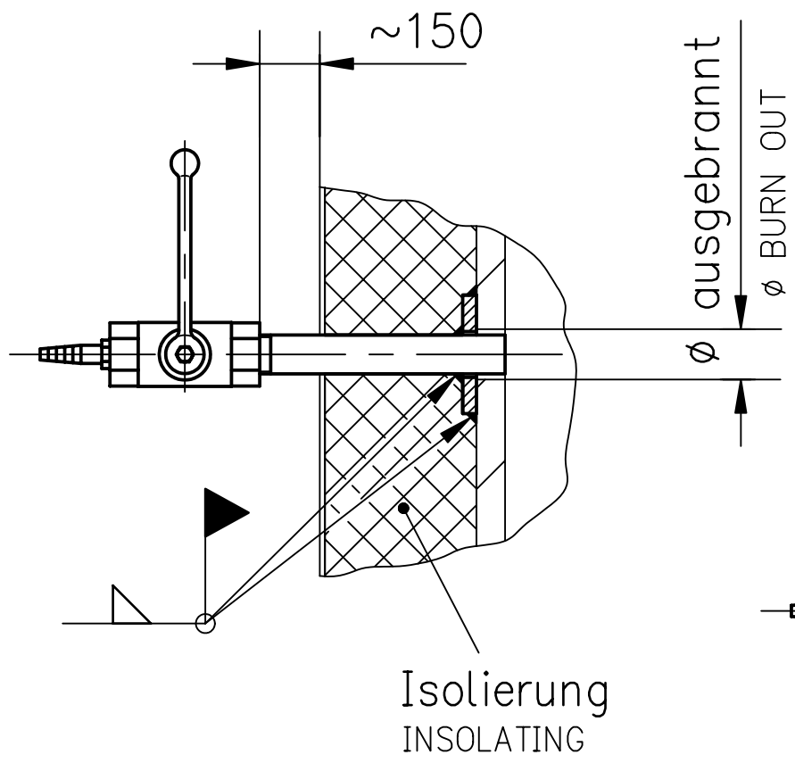
Schnitt C-C SECTION gedreht gezeichnet DRAWN TURNED
