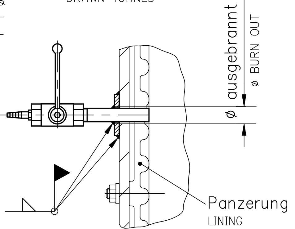
Schnitt D-D SECTION gedreht gezeichnet DRAWN TURNED
