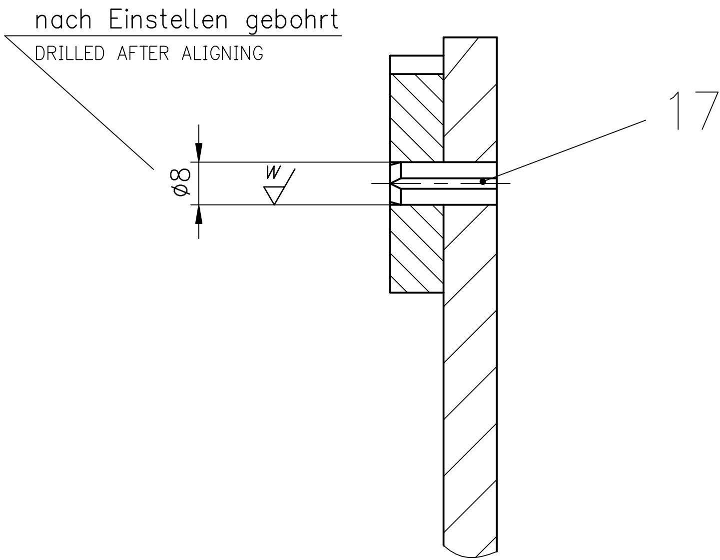
Schnitt A-A SECTION M1:1
