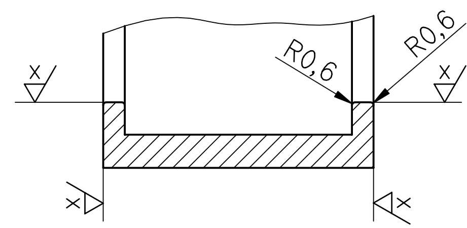
Einzelheit Z DETAIL M 1:1
