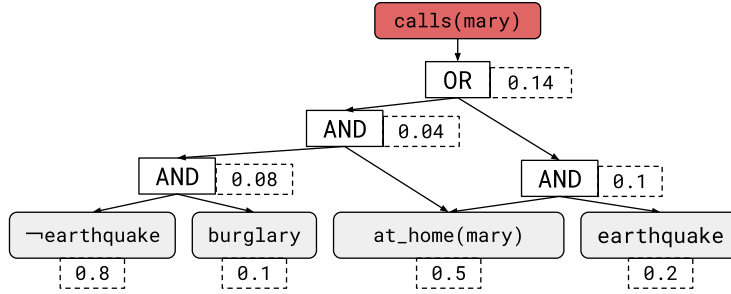
(d) The AC for query \text{calls}(\text{mary}) .
