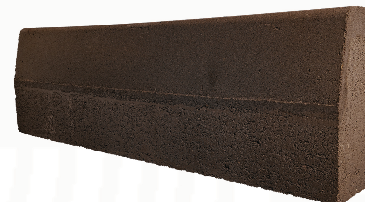
Curbstone 100*15*30 cm
