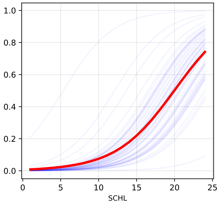
SCHL
