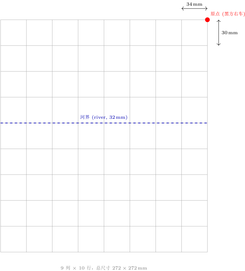
图 5.1: 棋盘几何与坐标映射示意。原点位于右上角（黑方右车），列间距 34 mm、普通行间距 30 mm、河界行间距 32 mm。
