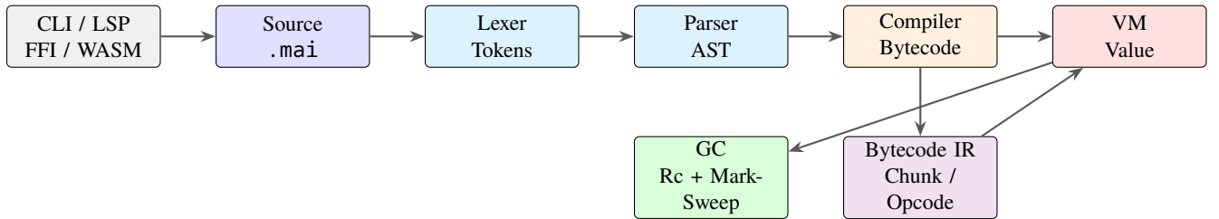
Figure 1: MaiLang 编译与执行流水线。上游为宿主集成层（CLI、LSP、FFI、WASM），下游为字节码 IR 与虚拟机，GC 跟踪运行时堆节点。
