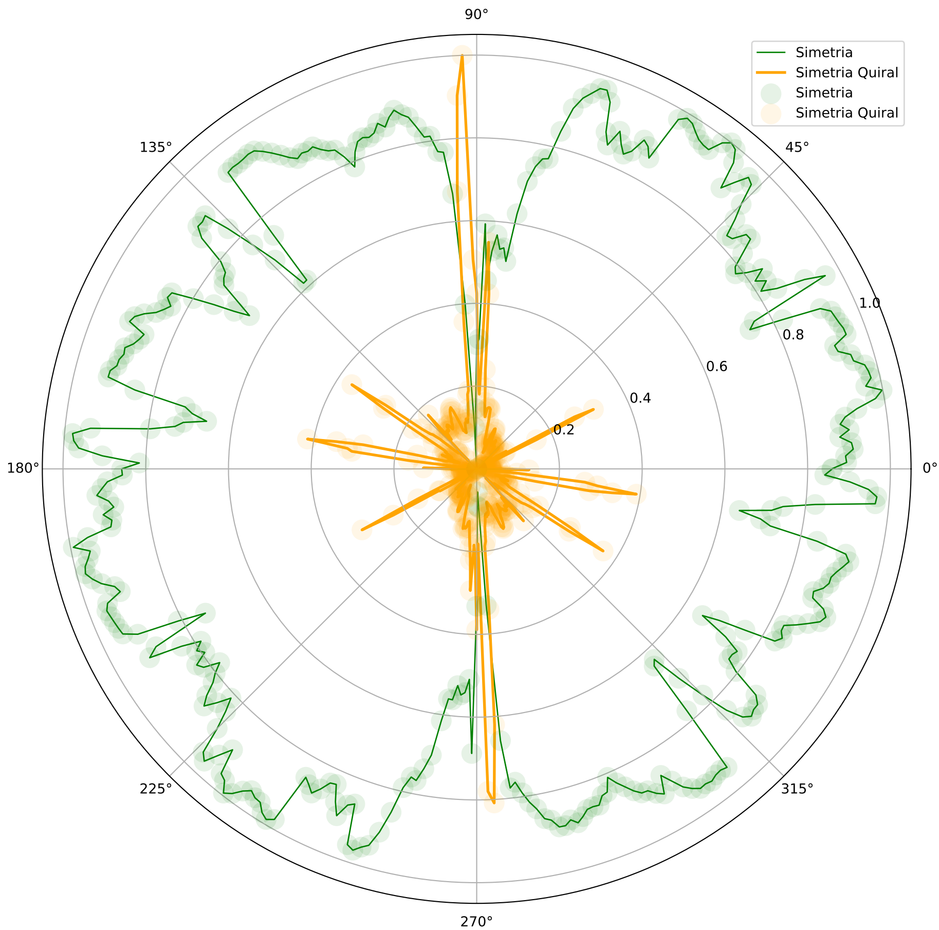
Comparação: Simetria vs. Simetria Quiral (Normalizadas)
