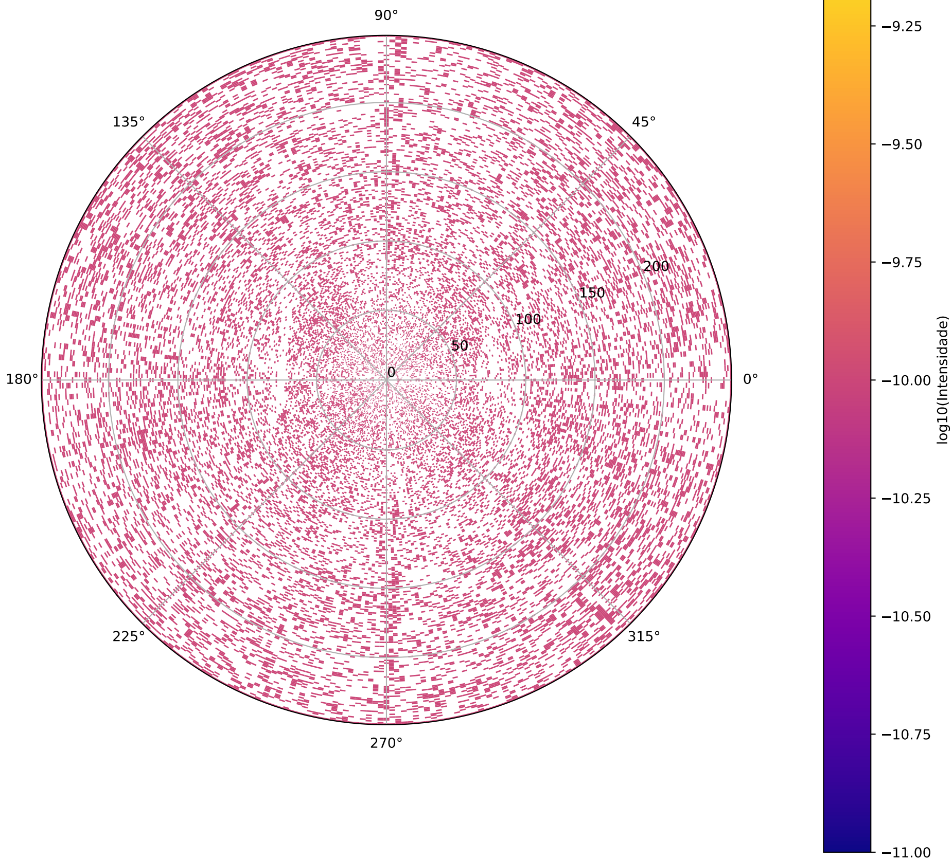
Operador Diferencial ( \hat{D} ) - Heatmap Polar (Escala Logarítmica)
