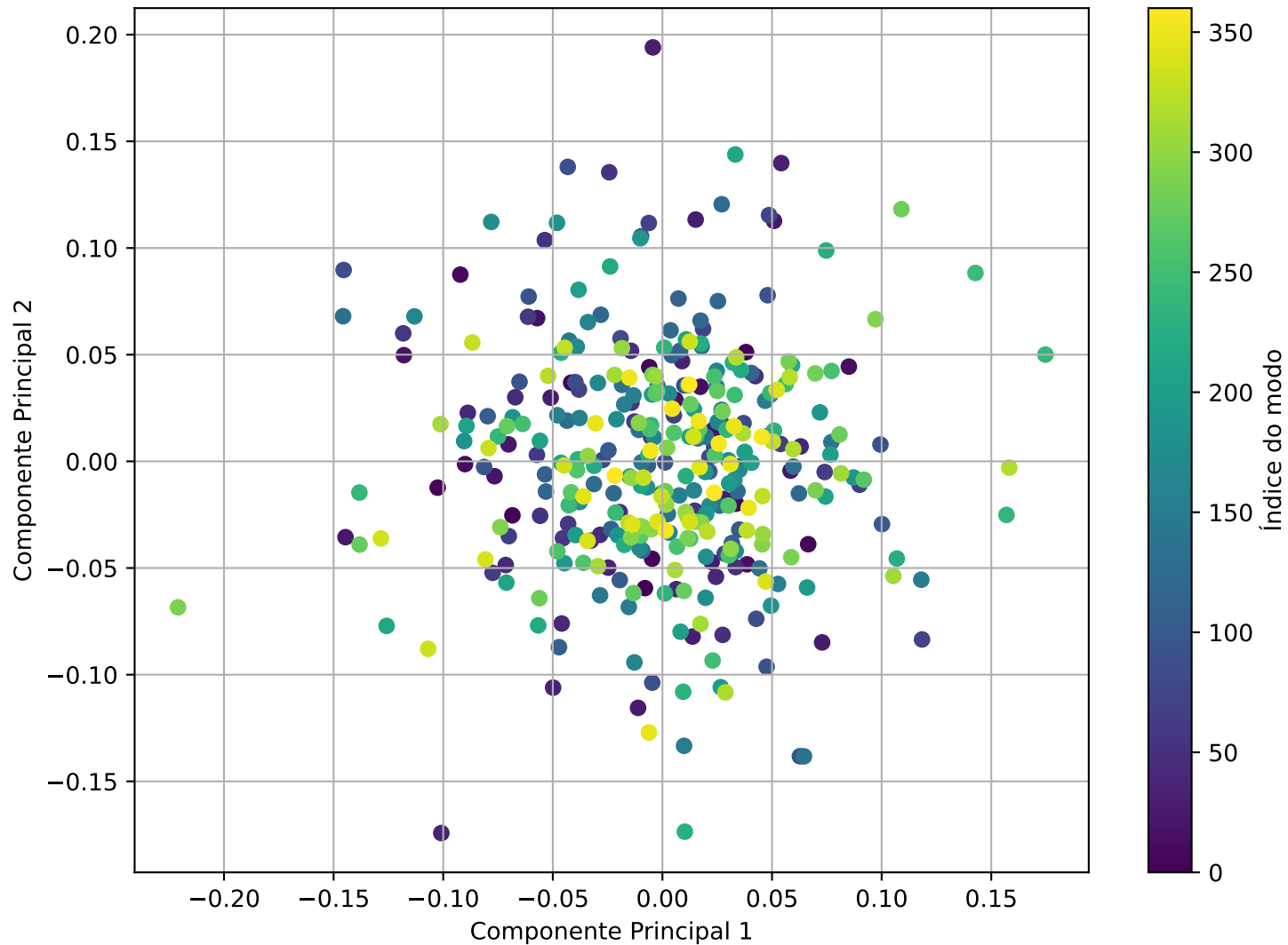
Projeção PCA dos Autoestados
