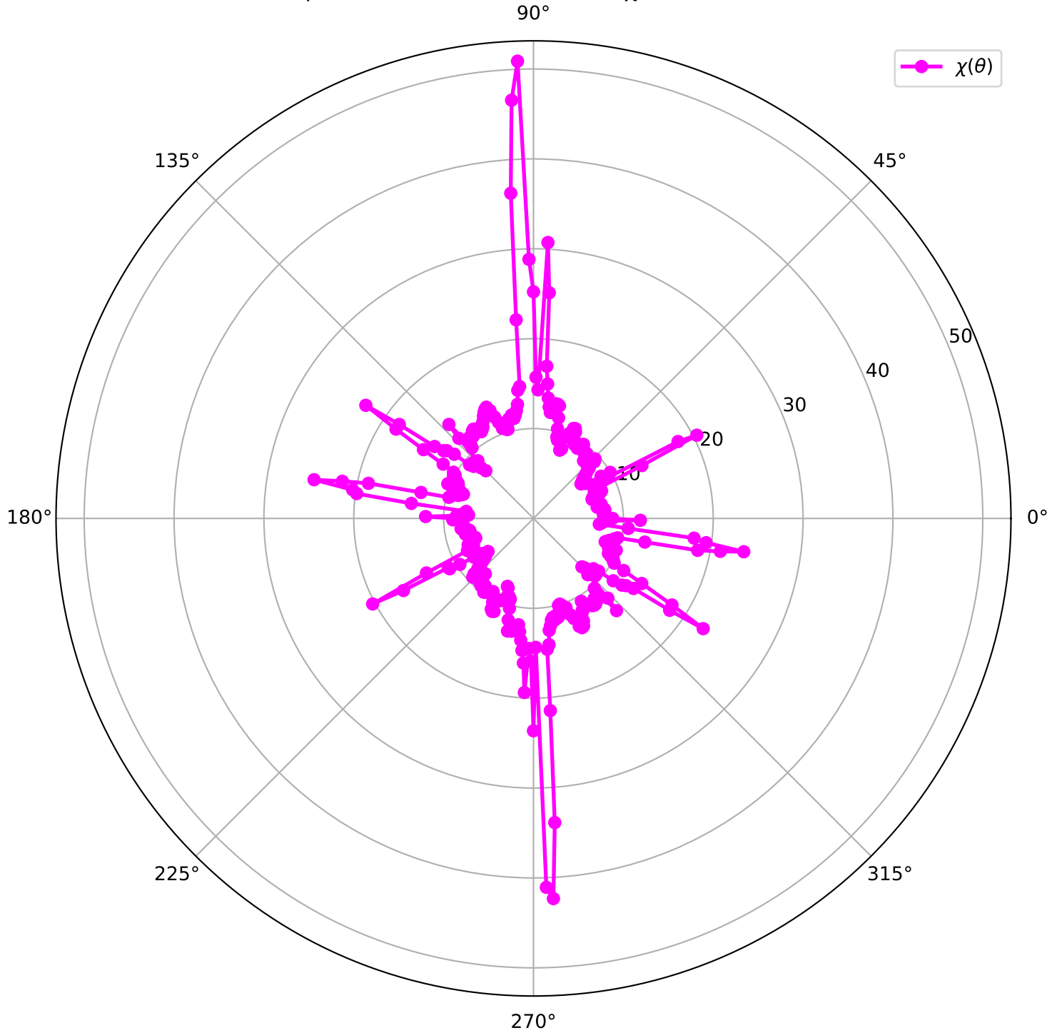
Operador de Simetria Quiral ( \chi ) - Plot Polar
