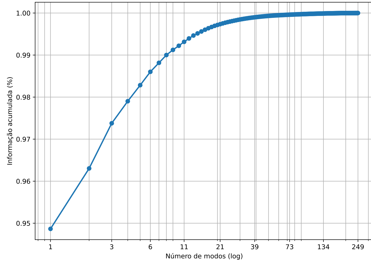
Informação Acumulada dos Modos
