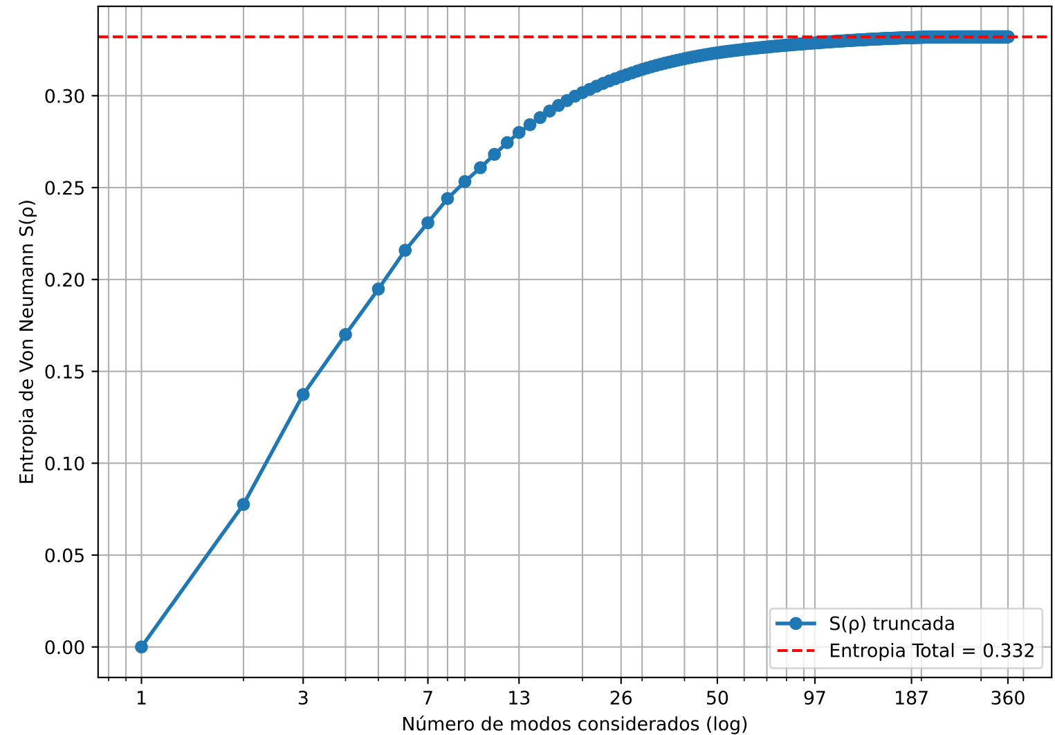
Entropia vs. Número de Modos
