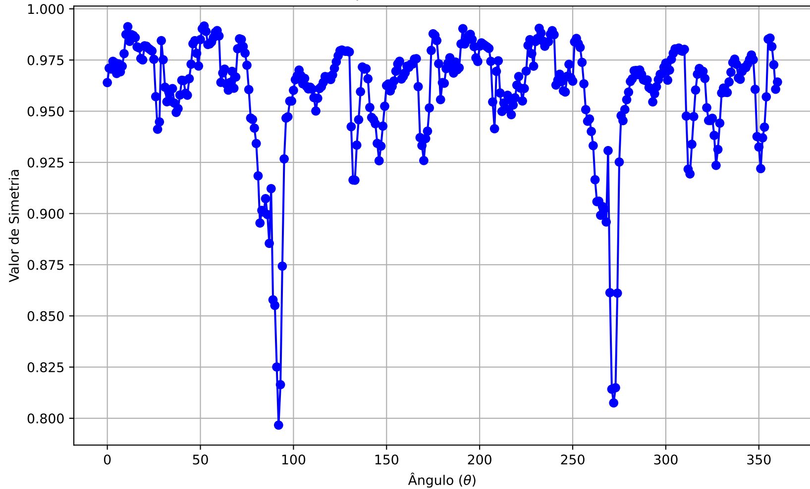
Operador de Simetria ( S )
