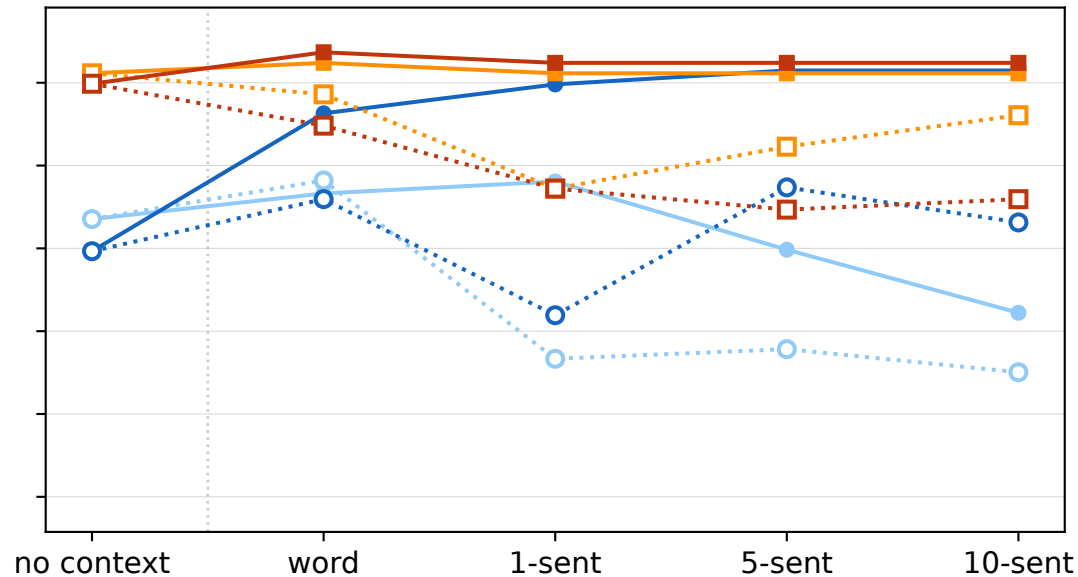
Phi-4-Multimodal
