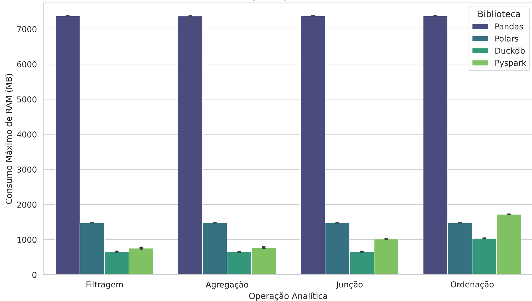
Consumo de RAM Pico (MB) por Operação - Dataset 1024MB (IC 95%)
