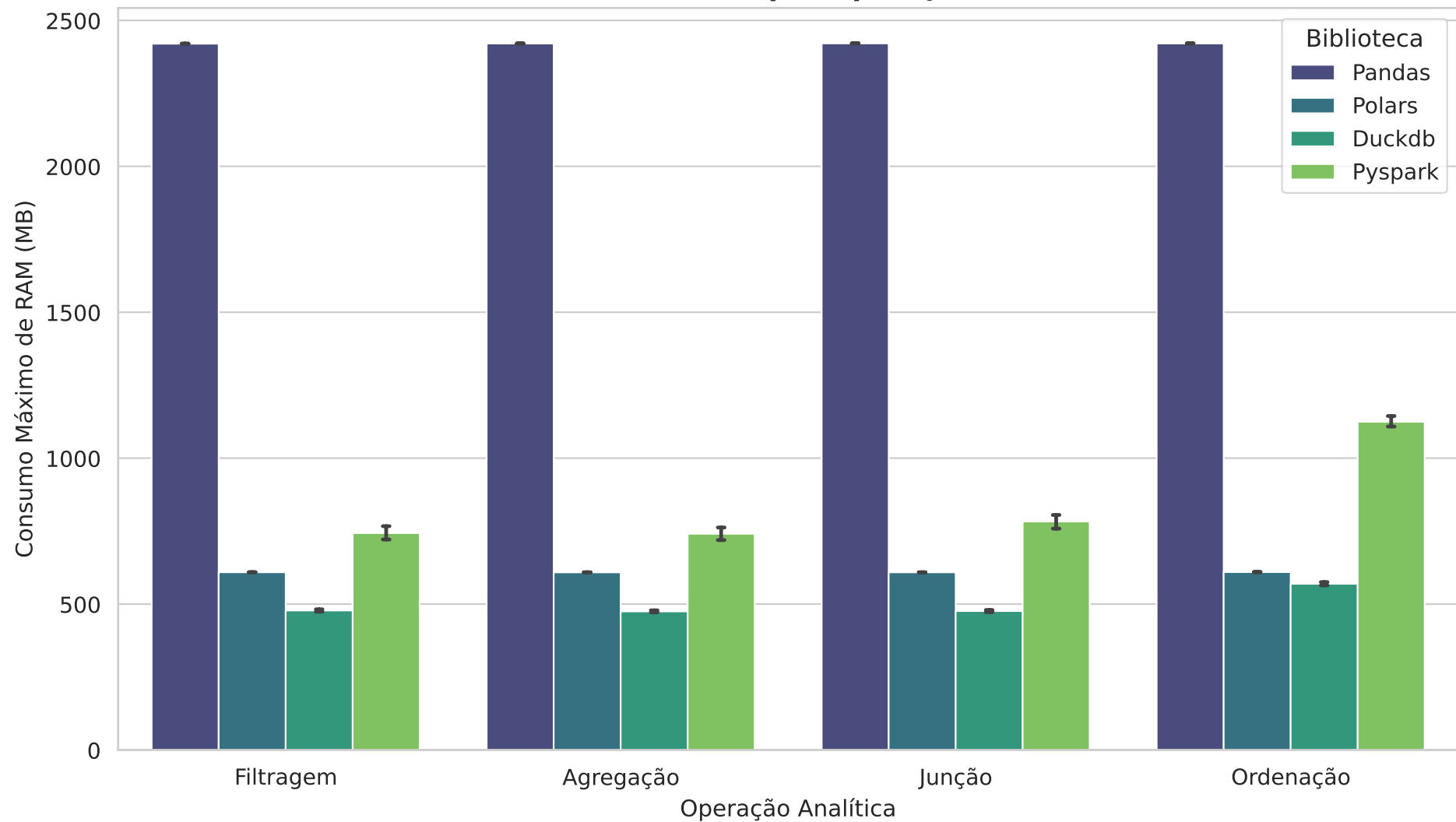
Consumo de RAM Pico (MB) por Operação - Dataset 256MB
